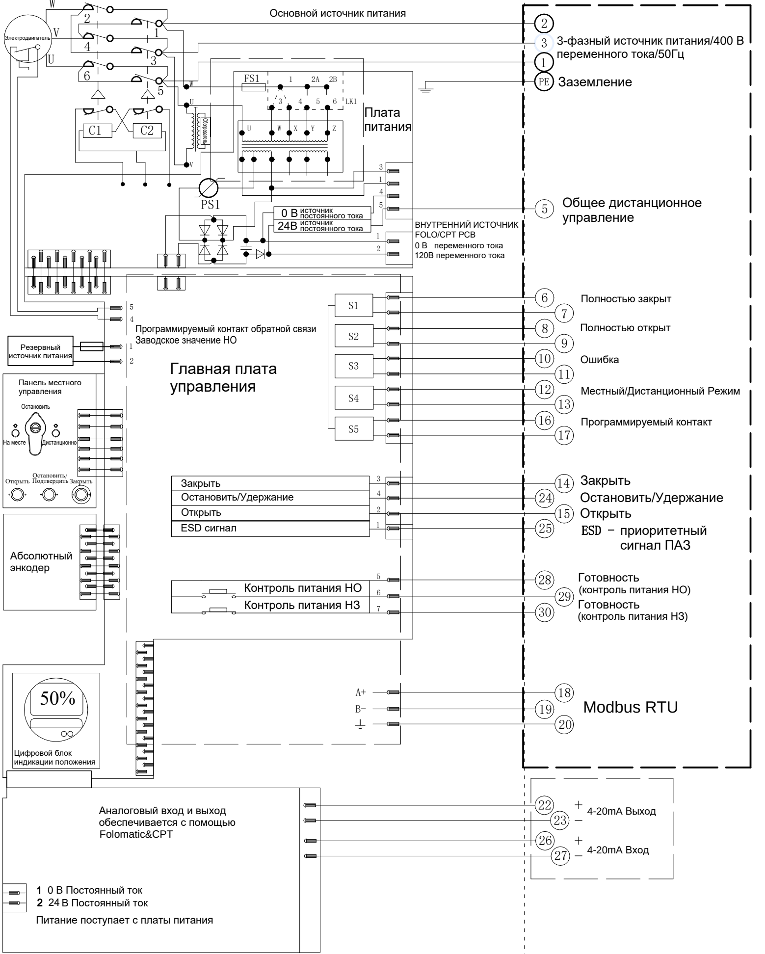
Электрическая схема №4-400B-24-6-MR-1 Серия SAL
