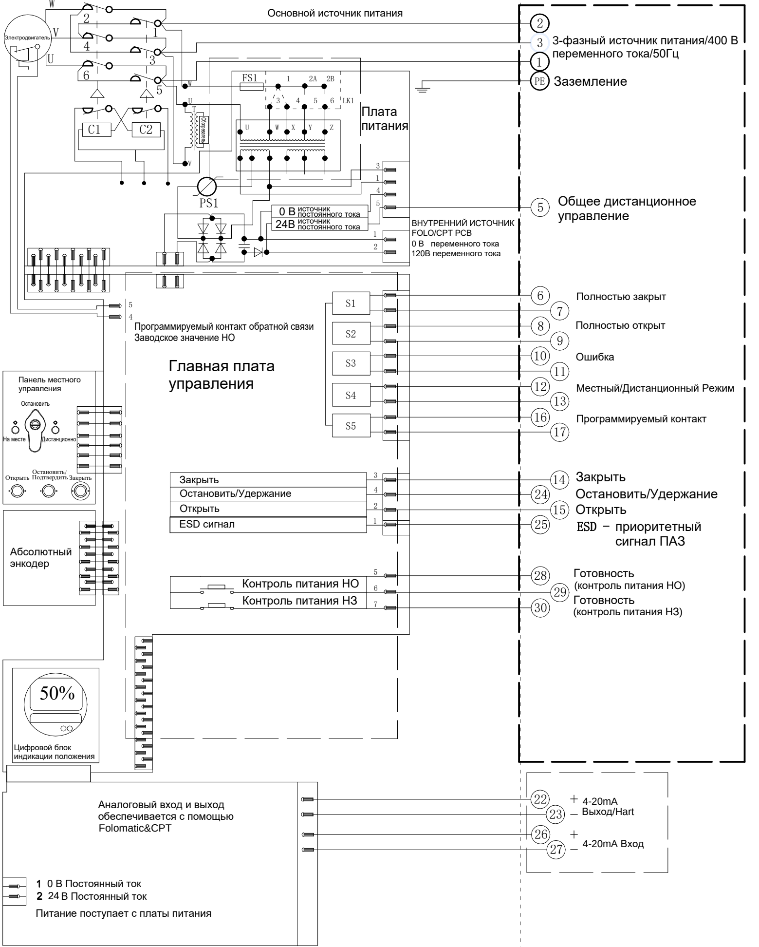
Электрическая схема №4-400-24-6-HR-1 Серия SAL
