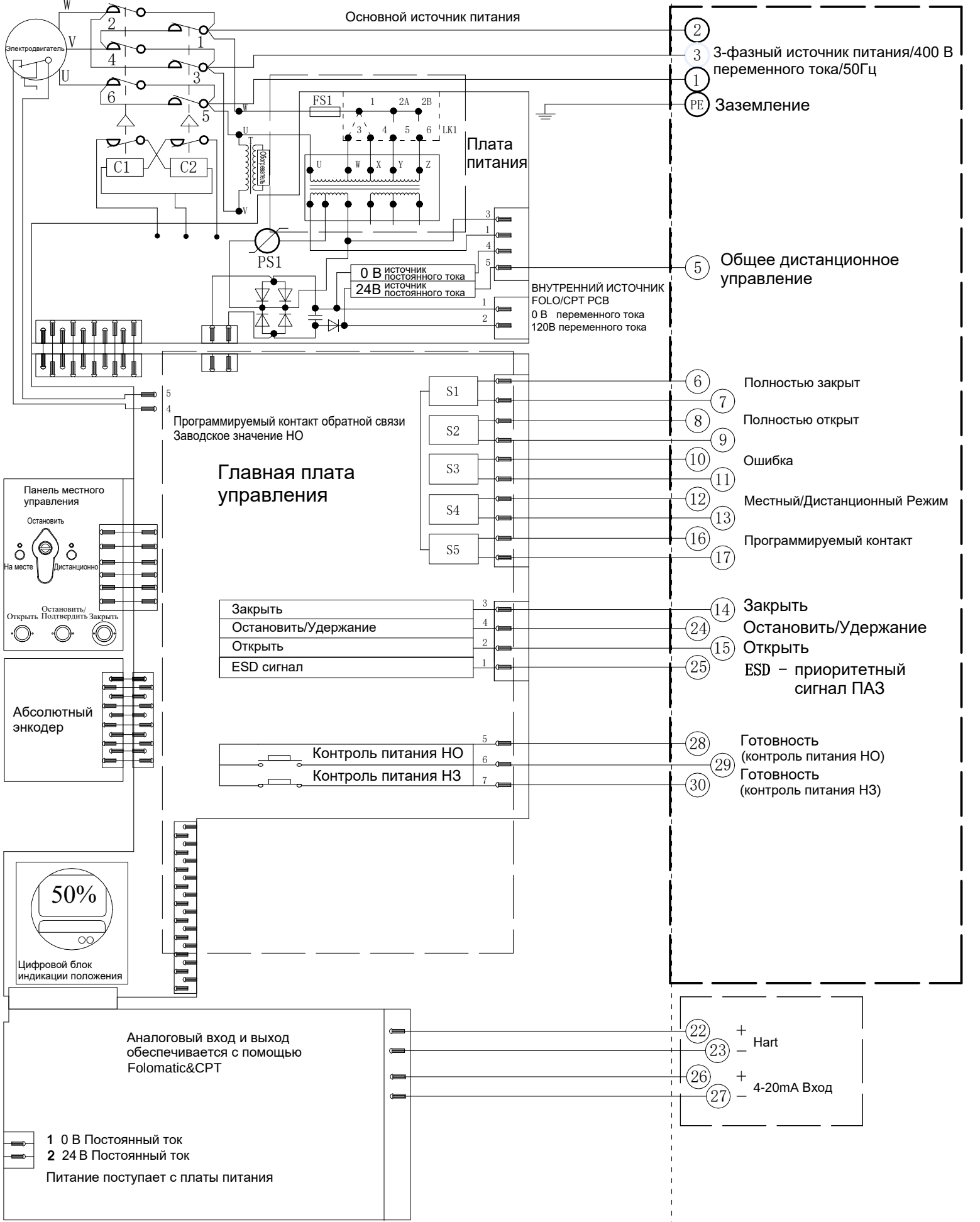
Электрическая схема №4-400-24-6-HR-2 Серия SAL
