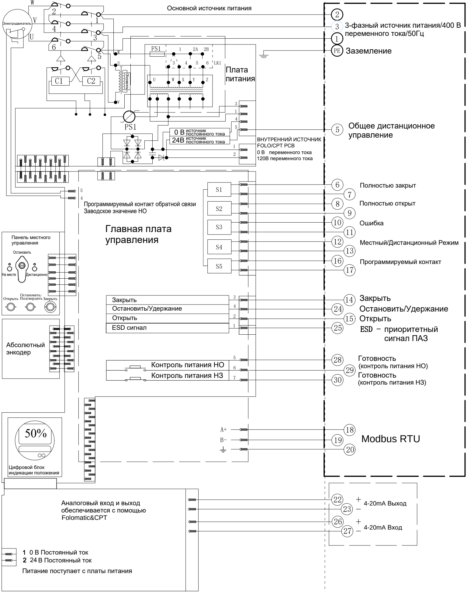
Электрическая схема №4-400-24-6-MR-1 Серия SAL
