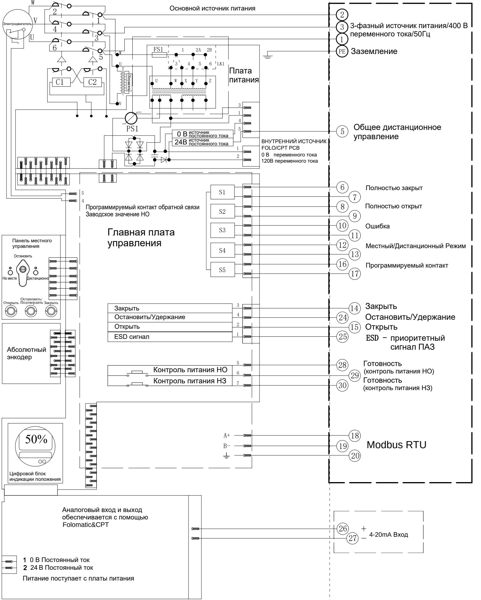
Электрическая схема №4-400-24-6-MR-2 Серия SAL
