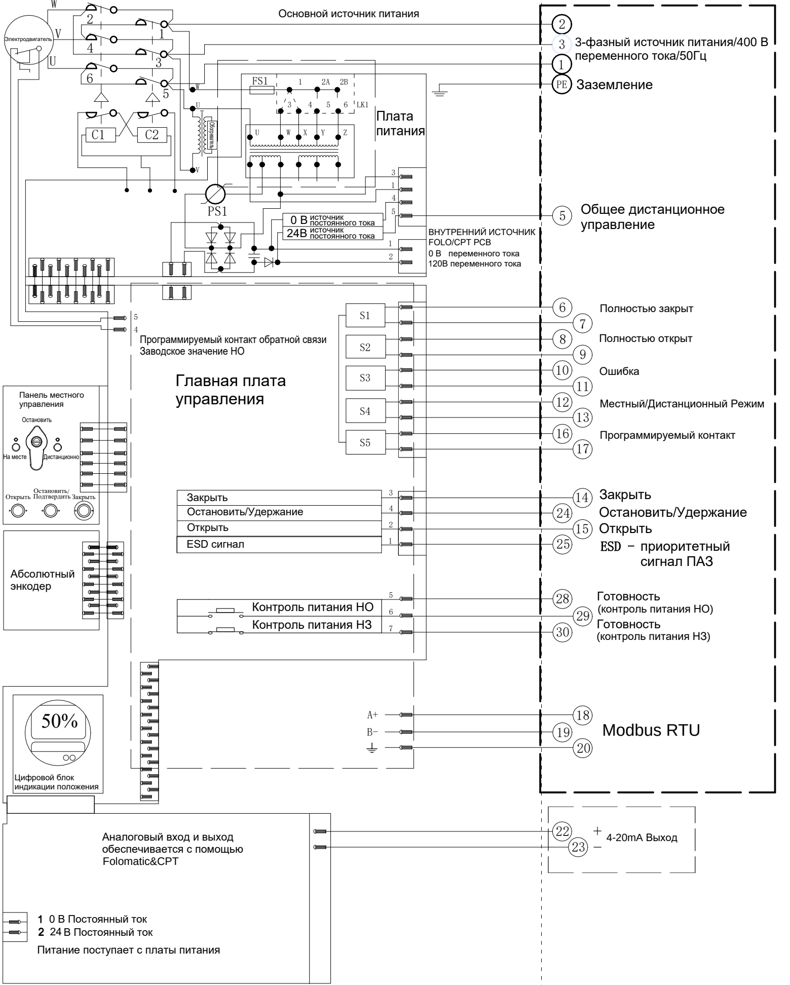
Электрическая схема №4-400-24-6-MR-3 Серия SAL
