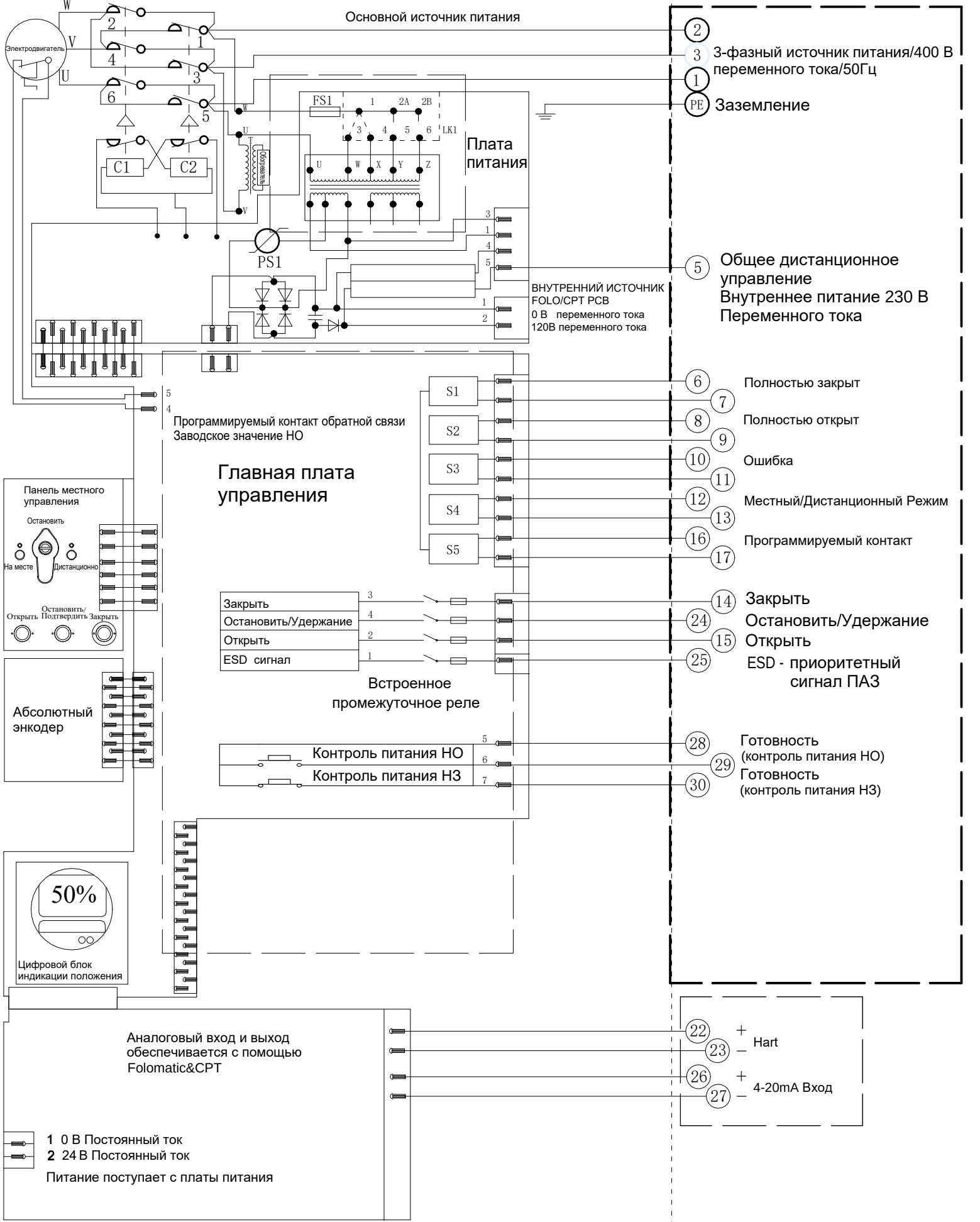
Электрическая схема №4-400-230-6-HR-2 Серия SAL
