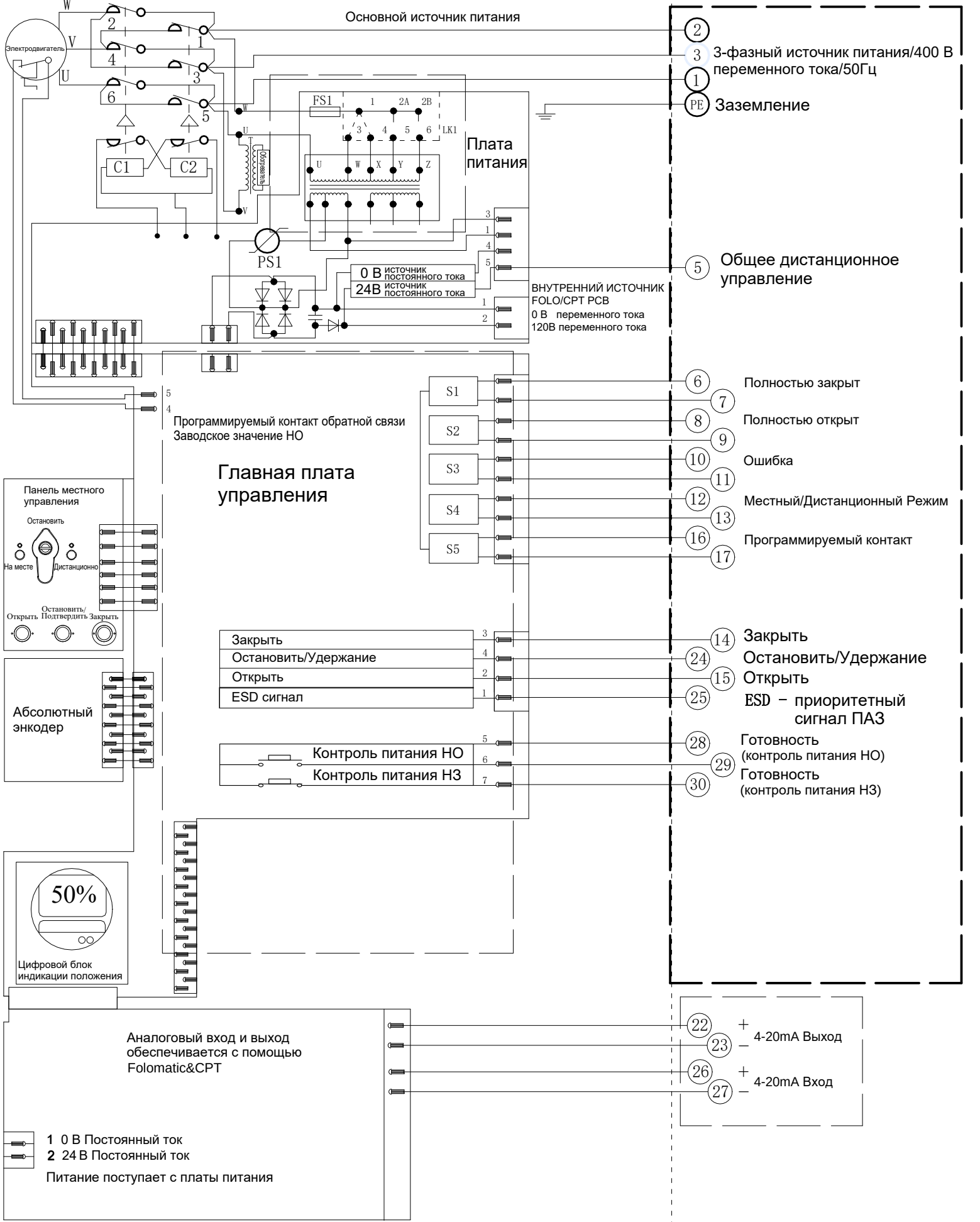
Электрическая схема №4-400-24-6-N-1 Серия SAL
