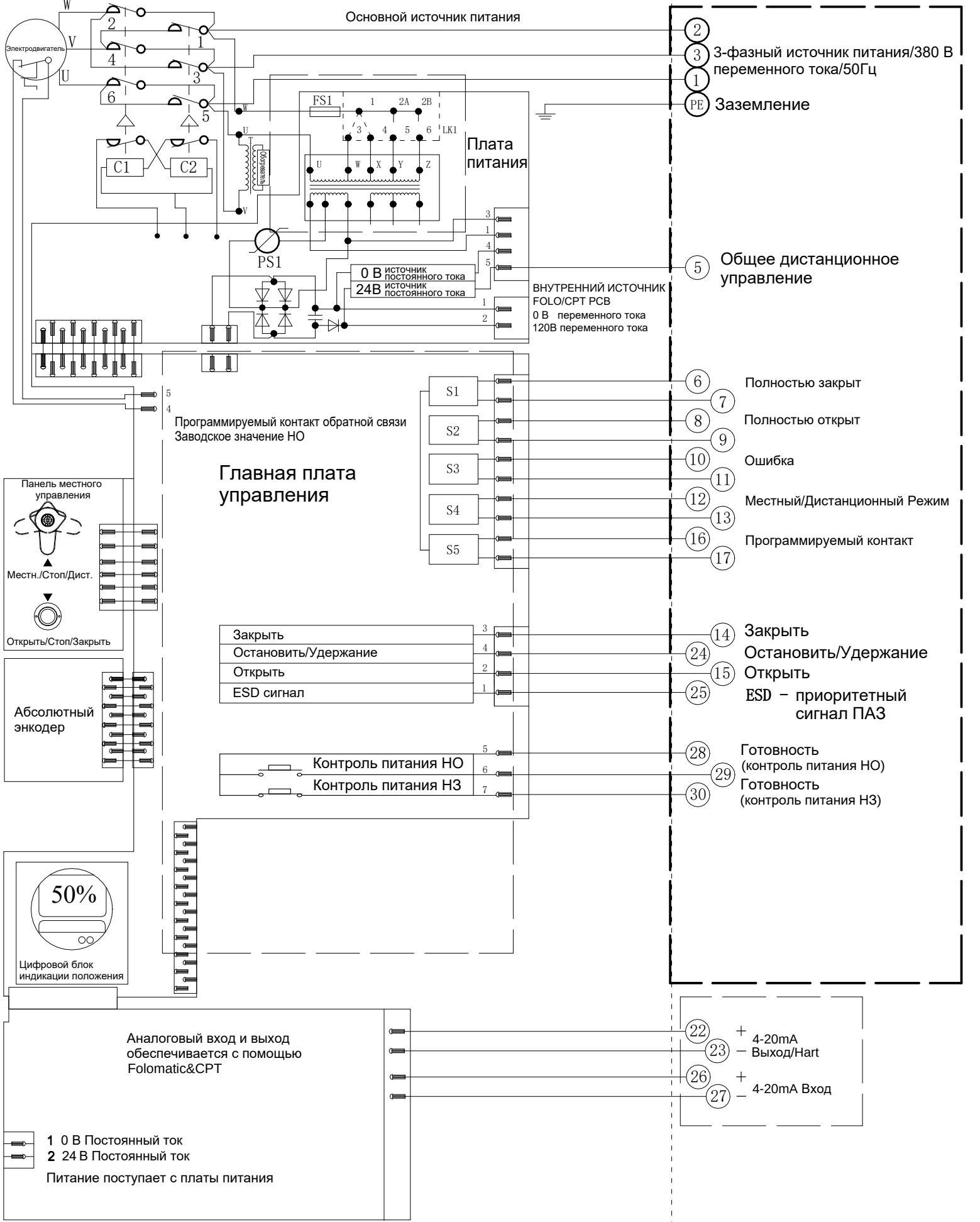
Электрическая схема №4-380-24-6-HR-1 Серия SAL
