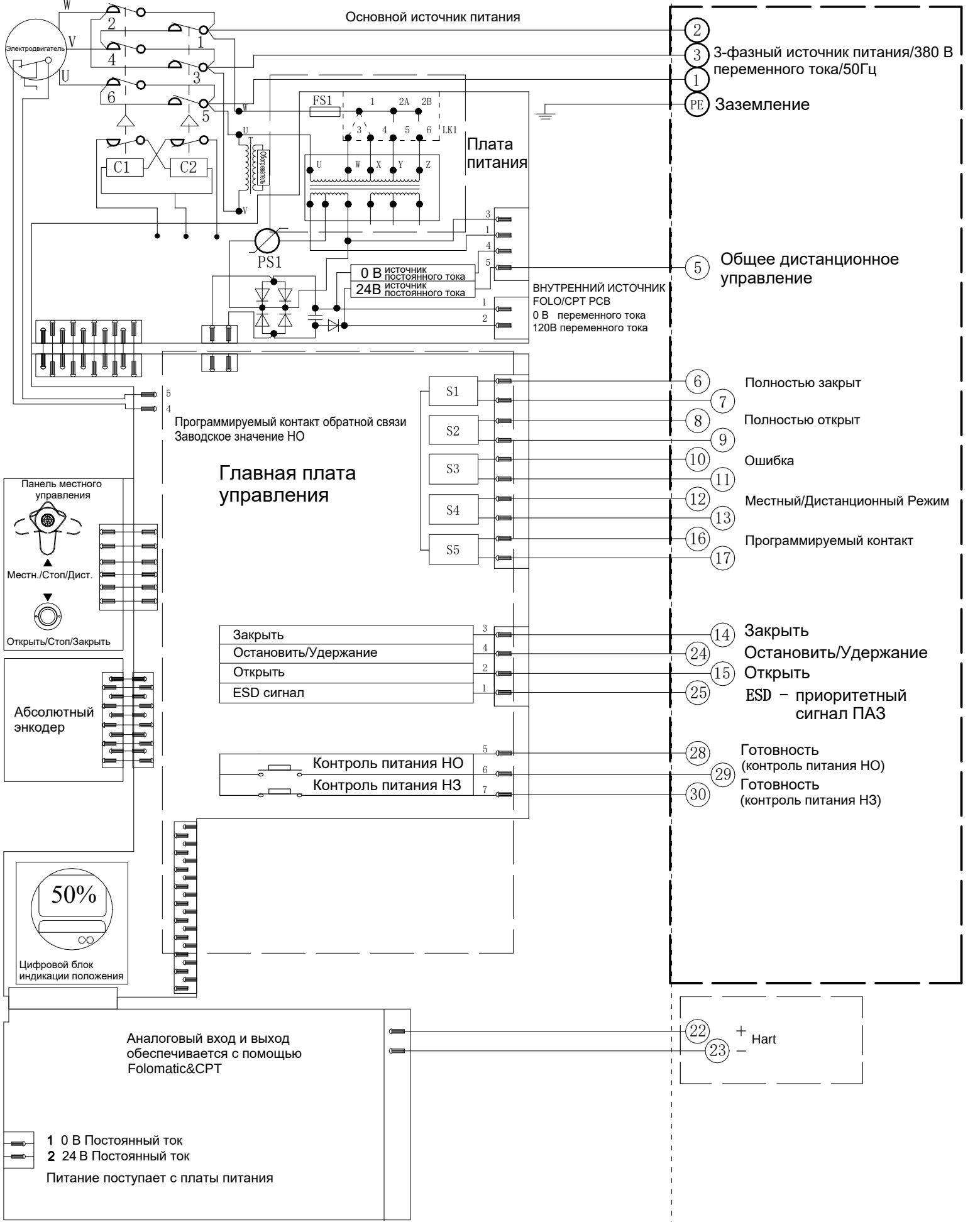
Электрическая схема №4-380-24-6-HR-0 Серия SAL
