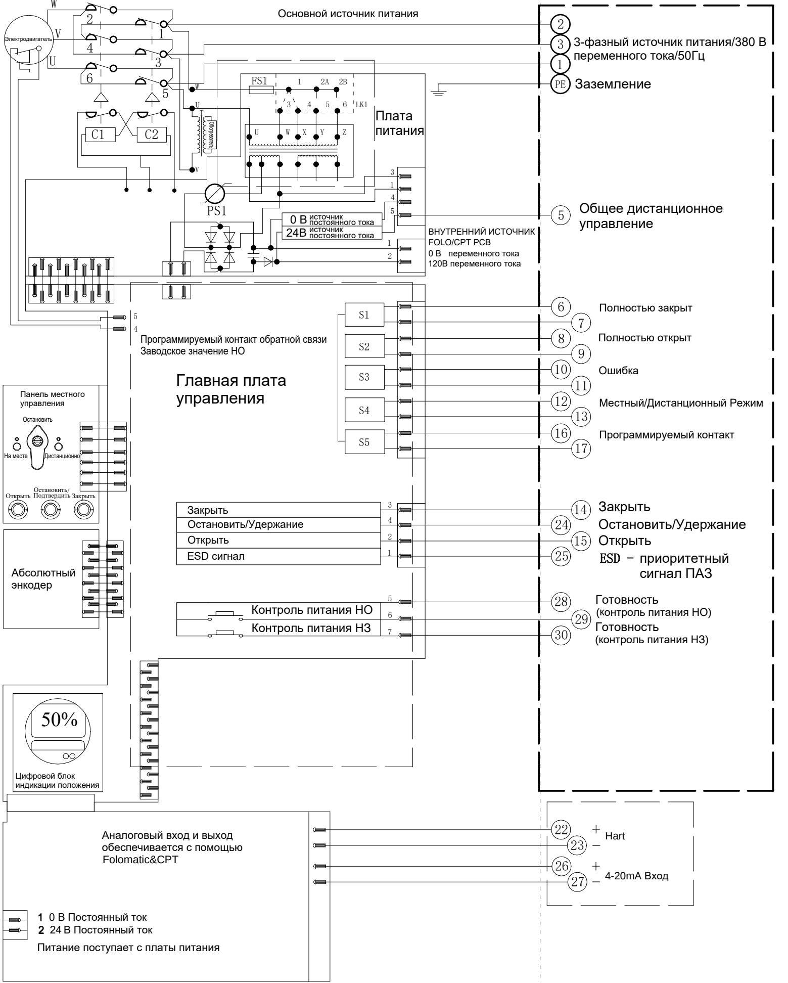
Электрическая схема №4-380-24-6-HR-2 Серия SAL
