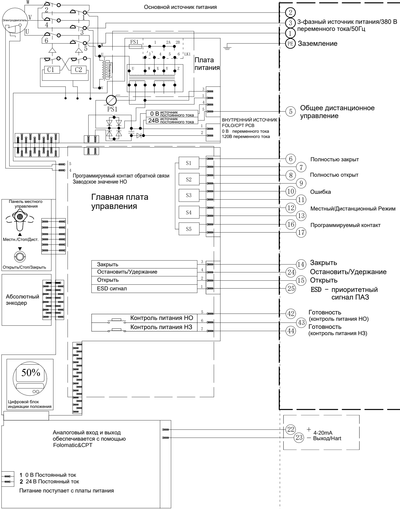
Электрическая схема №4-380-24-6-HR-3 Серия SAL
