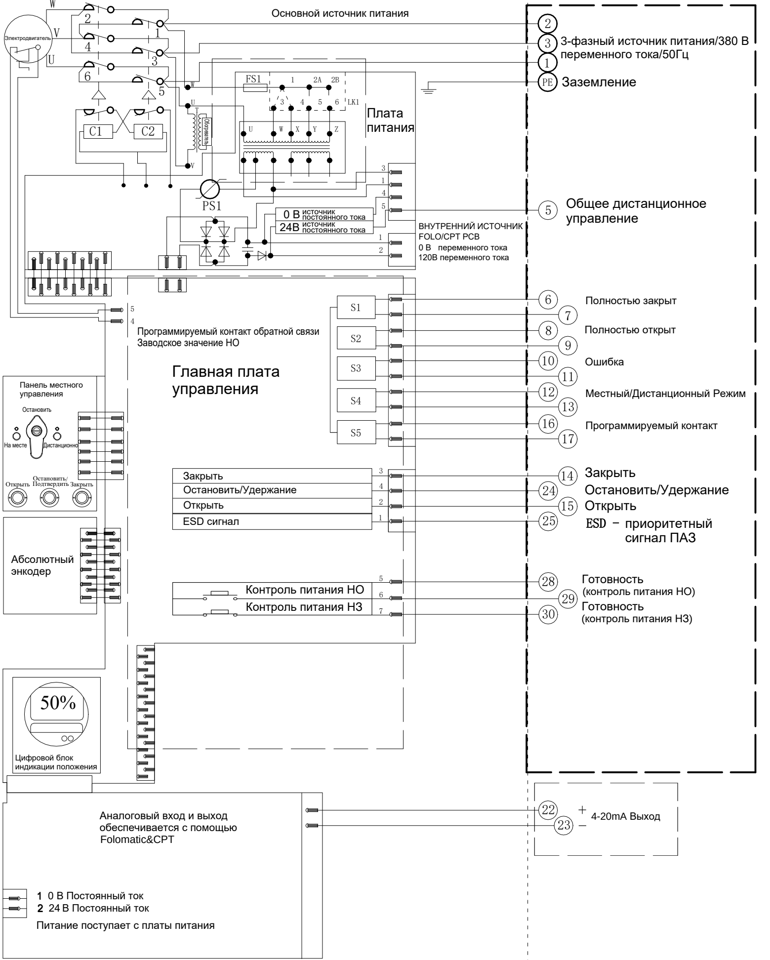
Электрическая схема №4-380-24-6-N-3 Серия SAL
