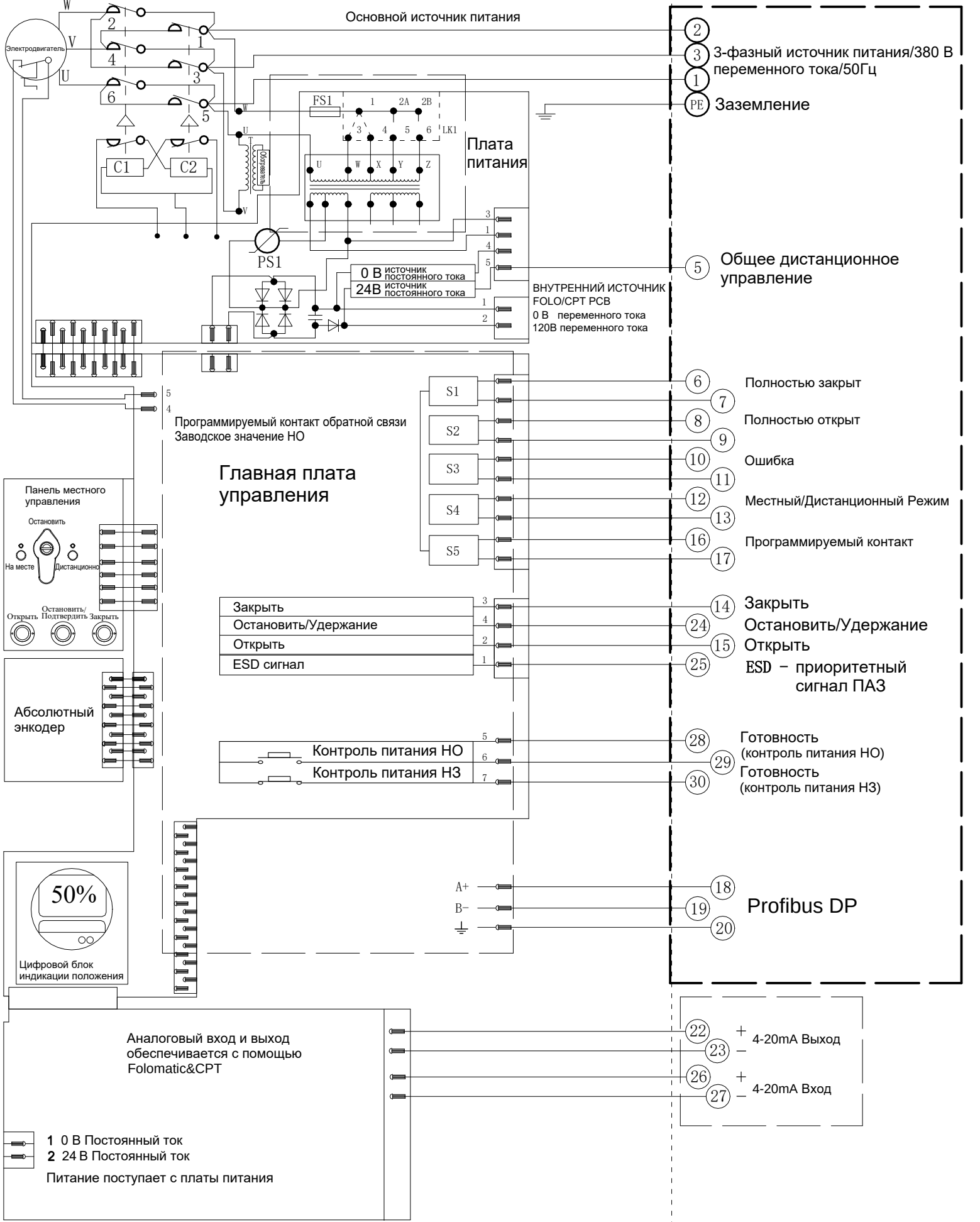
Электрическая схема №4-380-24-6-PR-1 Серия SAL
