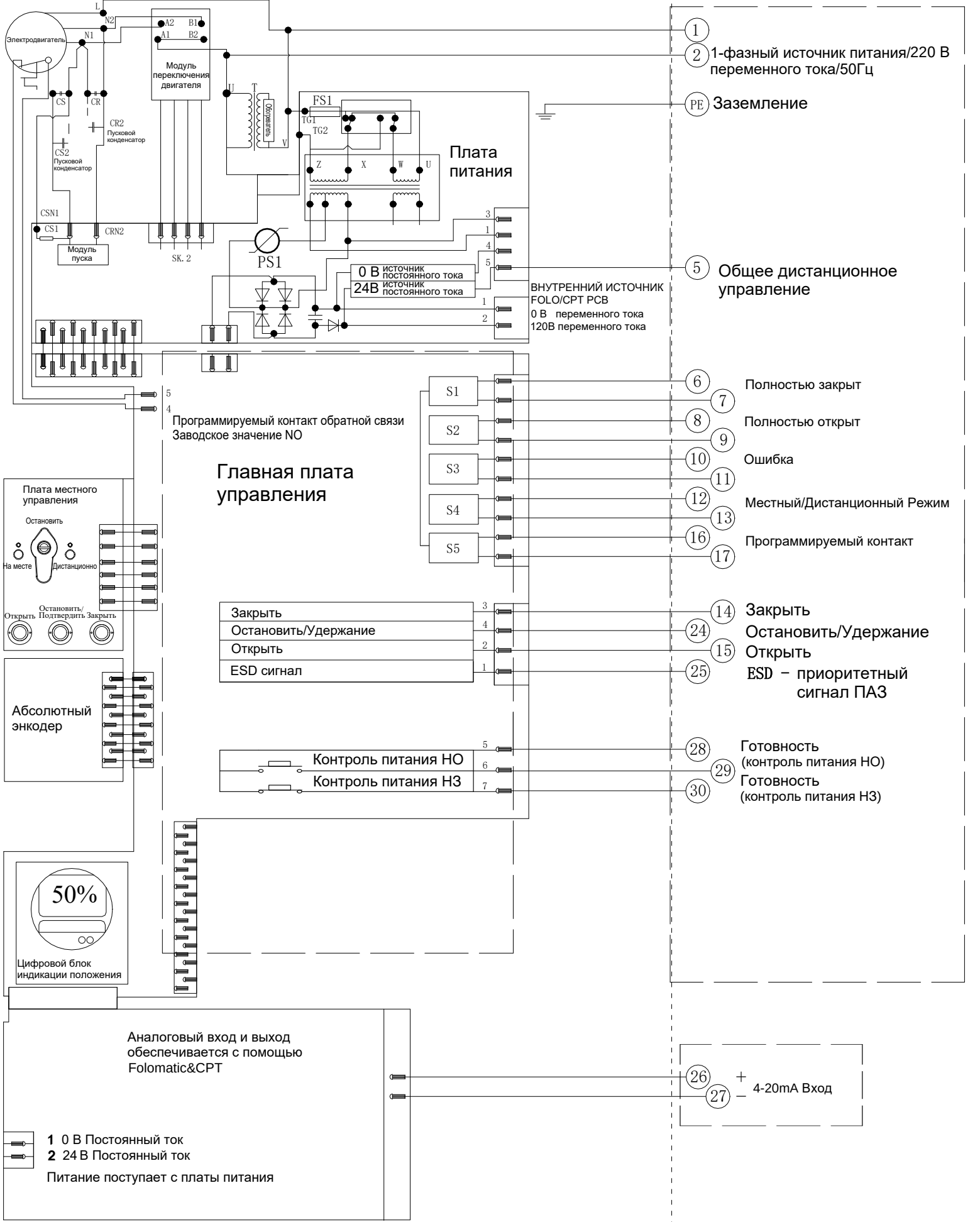
Электрическая схема 4-220-24-6-N-2 Серия SAL
