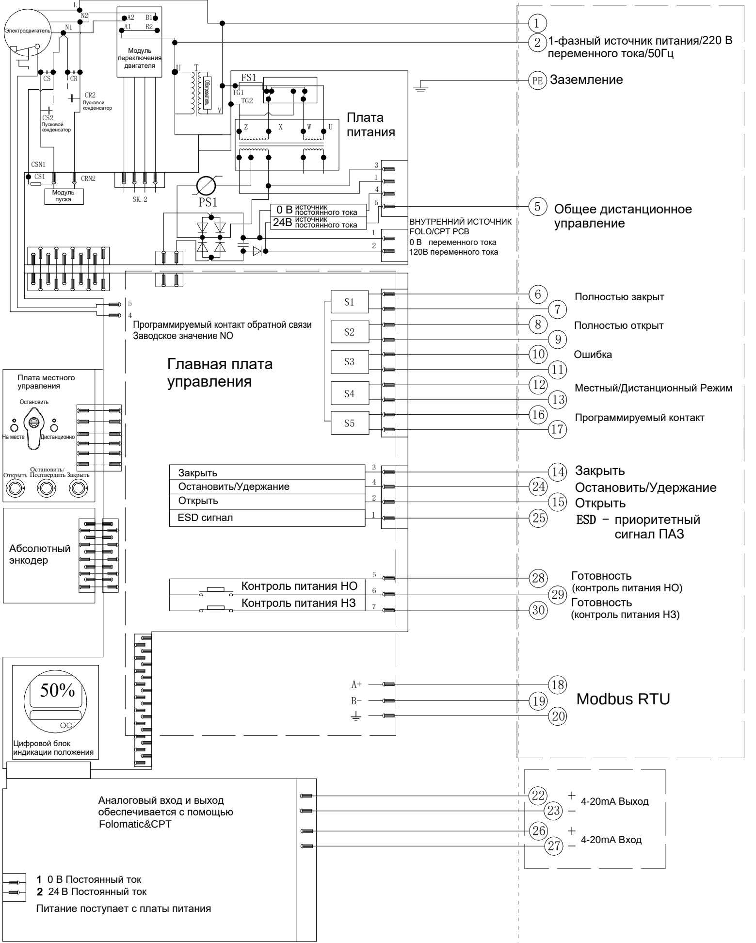
Электрическая схема 4-220-24-6-MR-1 Серия SAL
