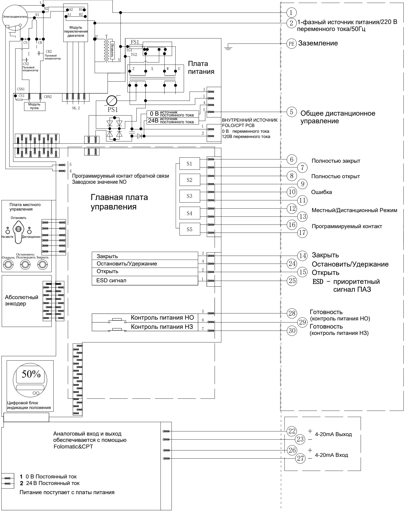
Электрическая схема 4-220-24-6-N-1 Серия SAL
