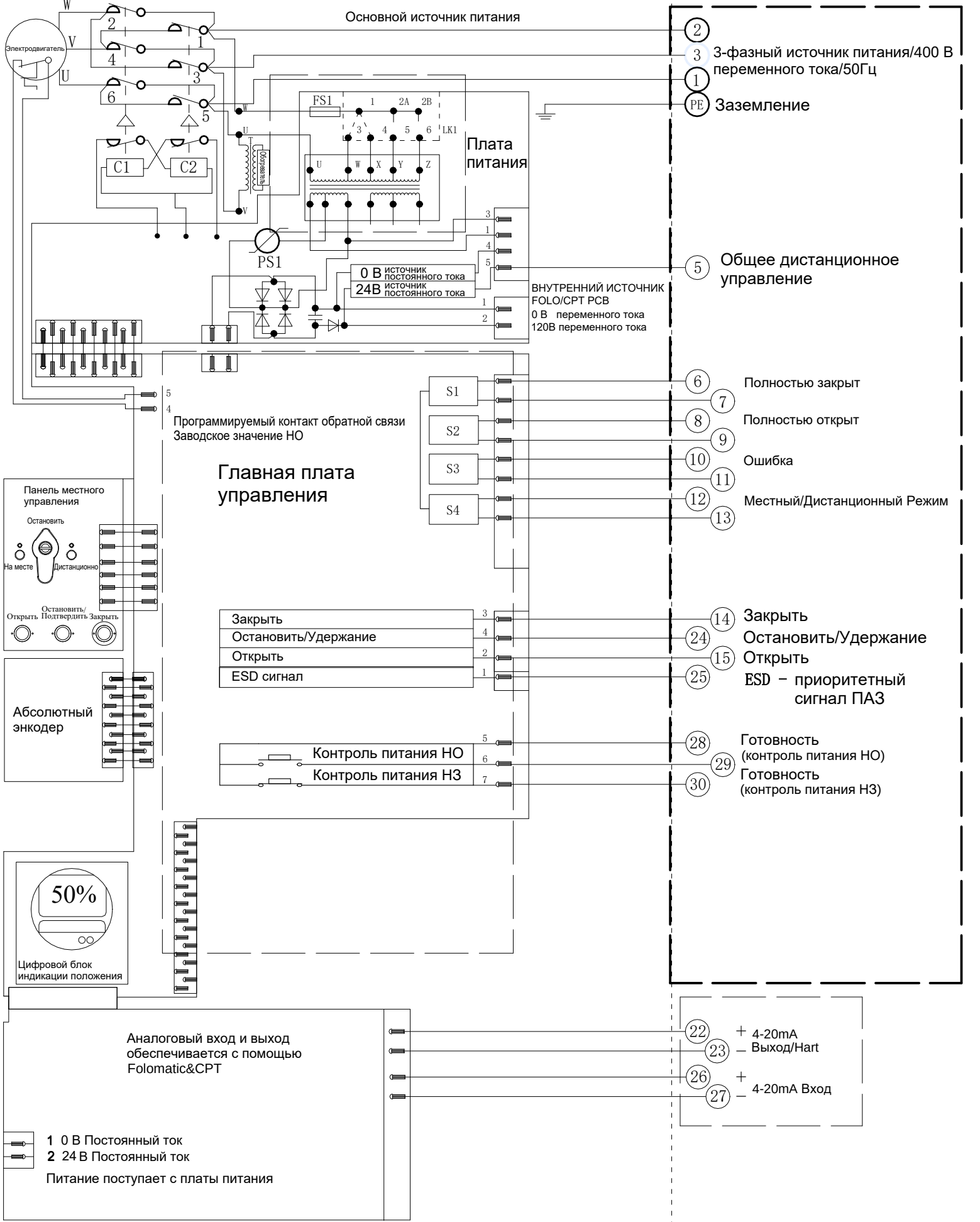
Электрическая схема №4-400-24-4-HR-1 Серия SAL
