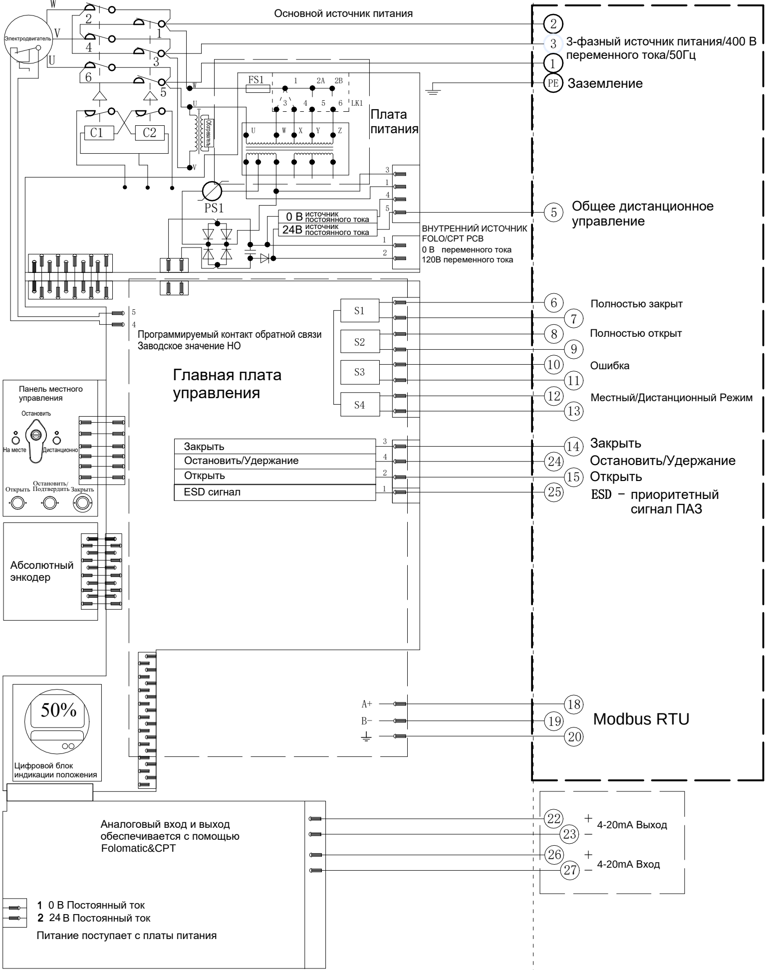
Электрическая схема №4-400-24-4-MR-1 Серия SAL
