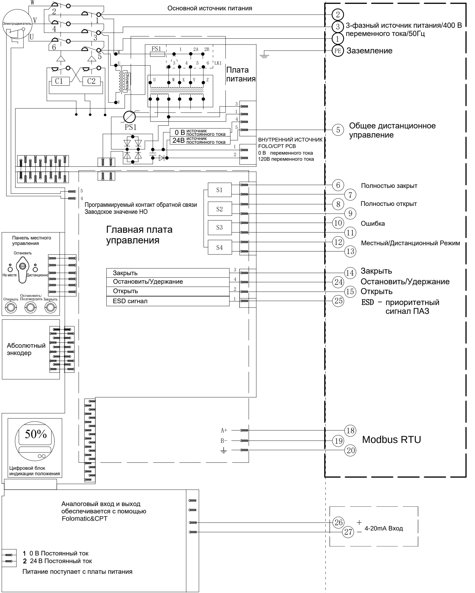
Электрическая схема №4-400-24-4-MR-2 Серия SAL
