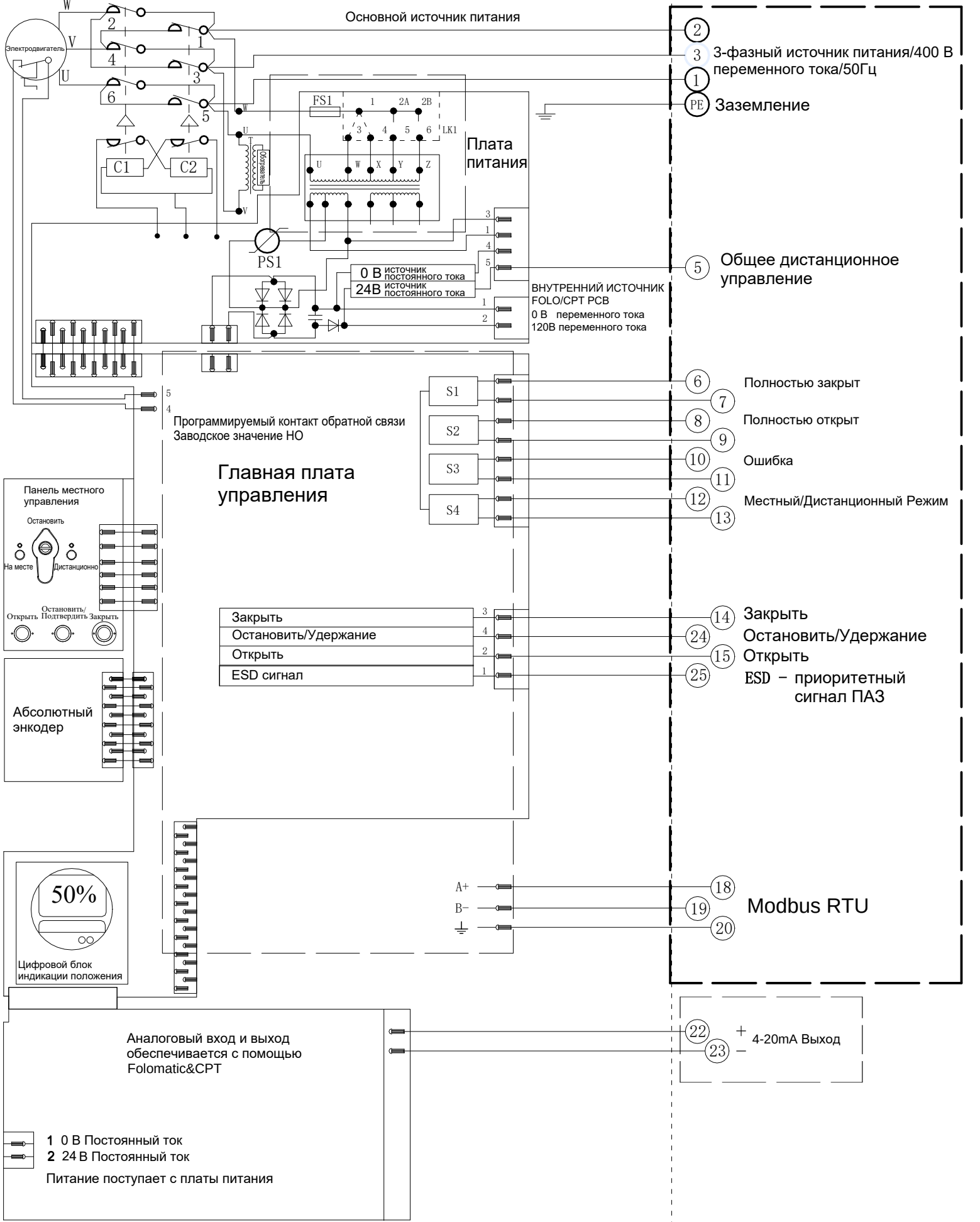
Электрическая схема №4-400-24-4-MR-3 Серия SAL
