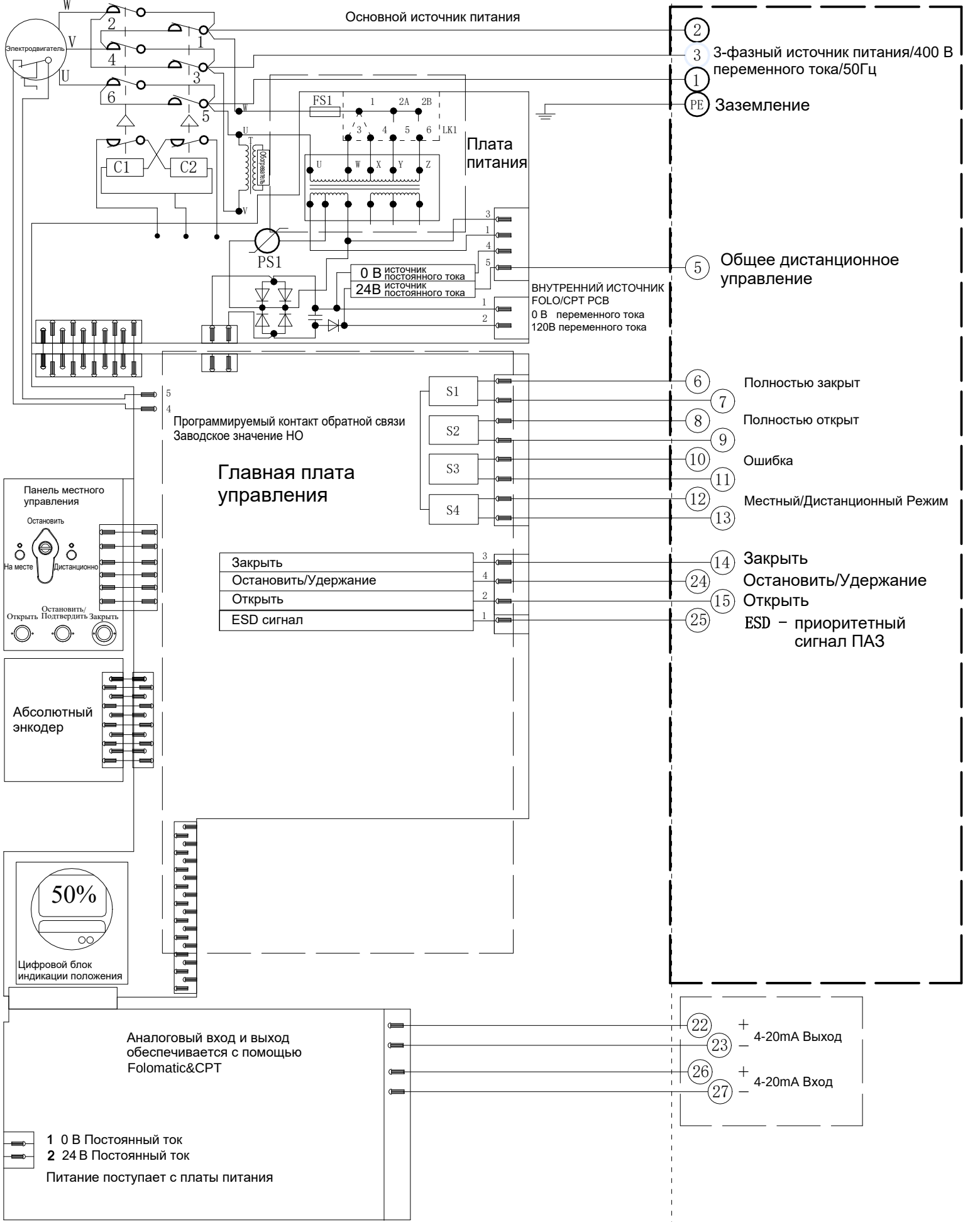
Электрическая схема №4-400-24-4-N-1 Серия SAL
