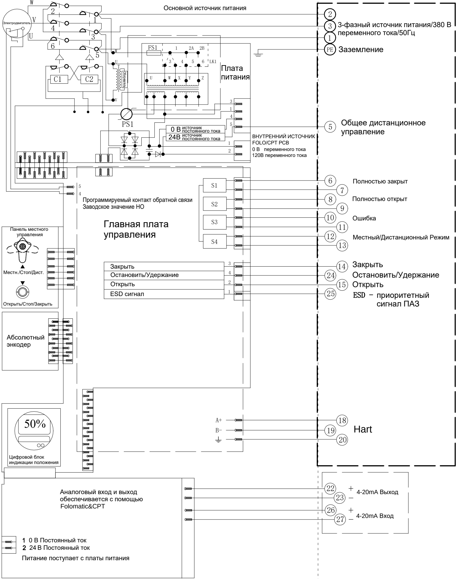
Электрическая схема №4-380-24-4-HR-1 Серия SAL
