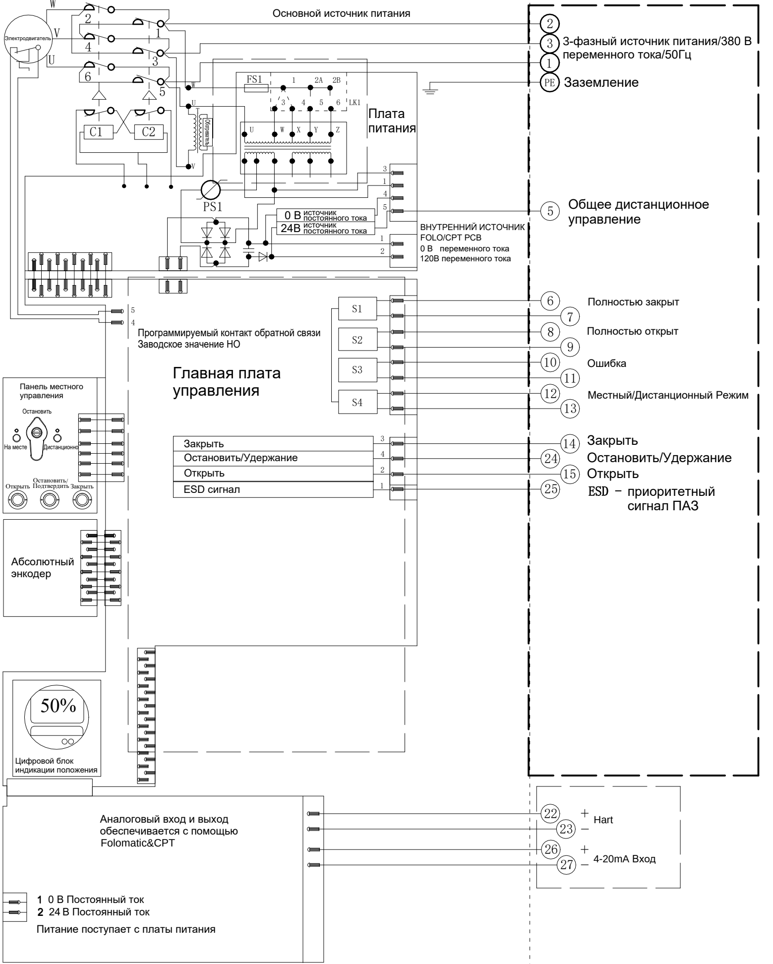
Электрическая схема №4-380-24-4-HR-2 Серия SAL
