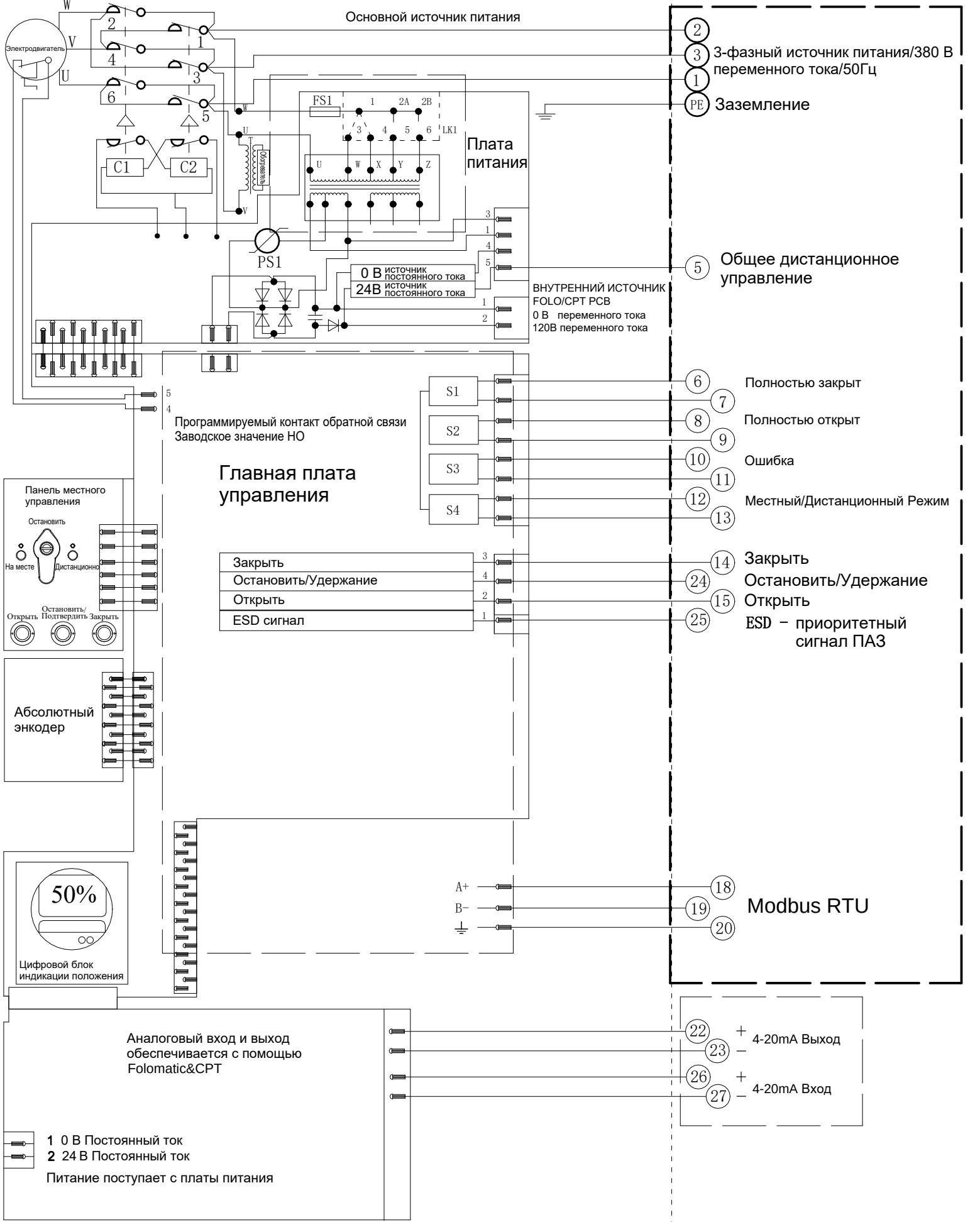
Электрическая схема №4-380-24-4-MR-1 Серия SAL
