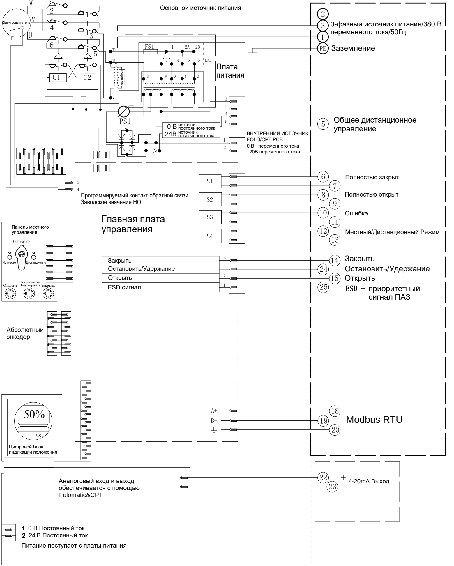
Электрическая схема №4-380-24-4-MR-3 Серия SAL
