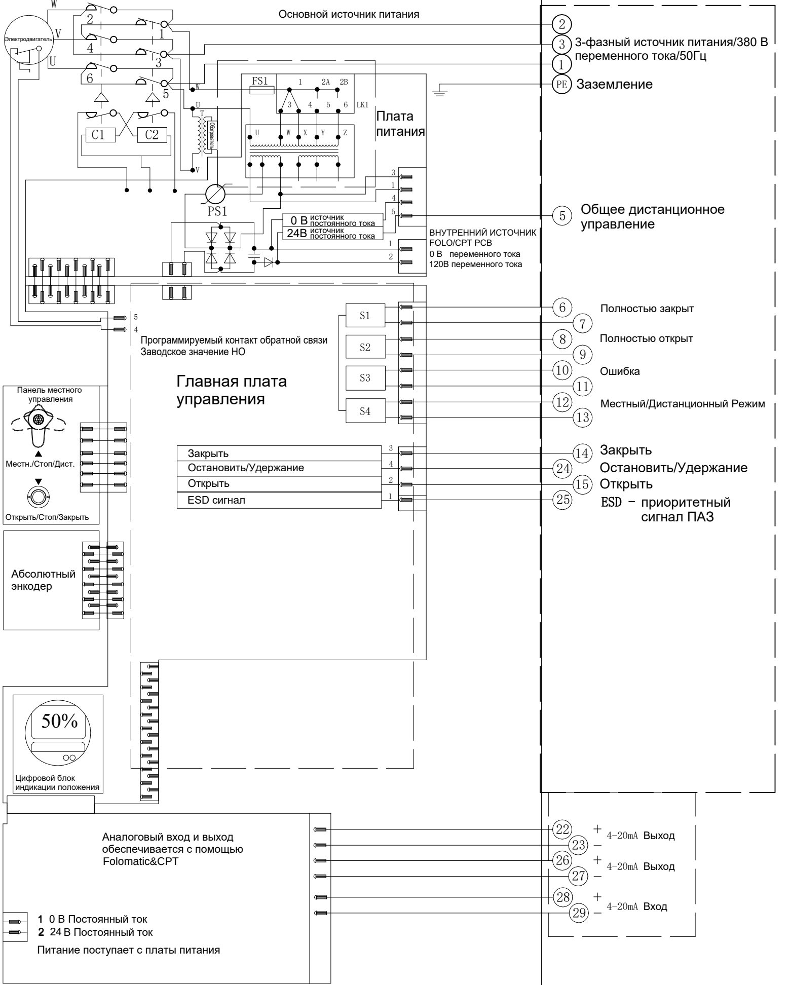
Электрическая схема №4-380-24-4-N-5 Серия SAL
