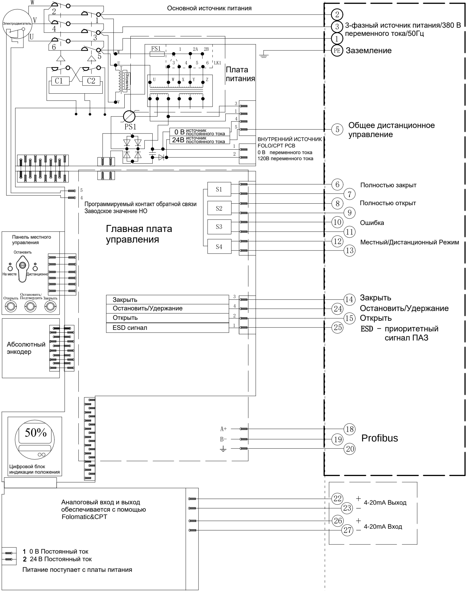
Электрическая схема №4-380-24-4-PR-1 Серия SAL
