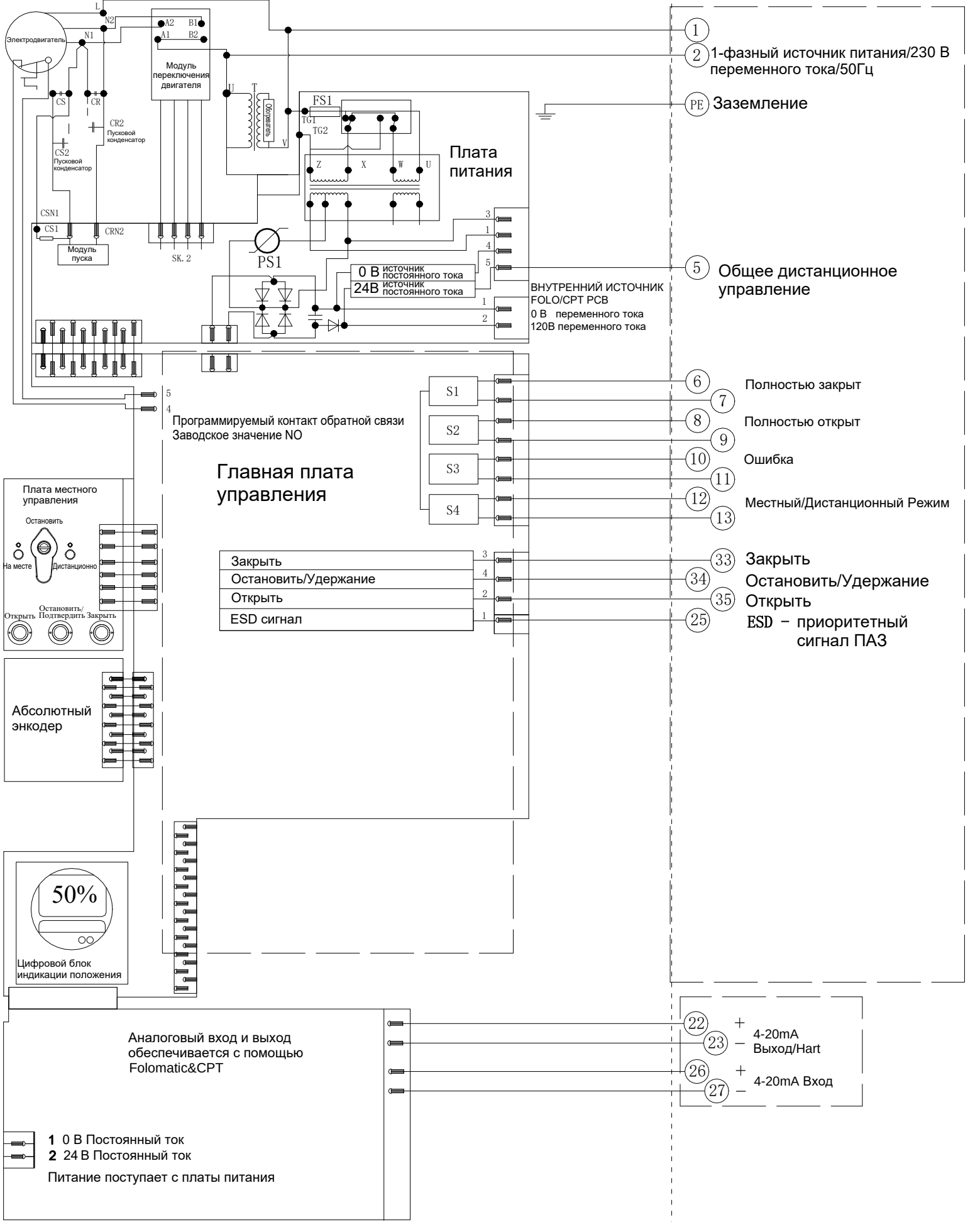
Электрическая схема 4-230-24-4-HR-1 Серия SAL
