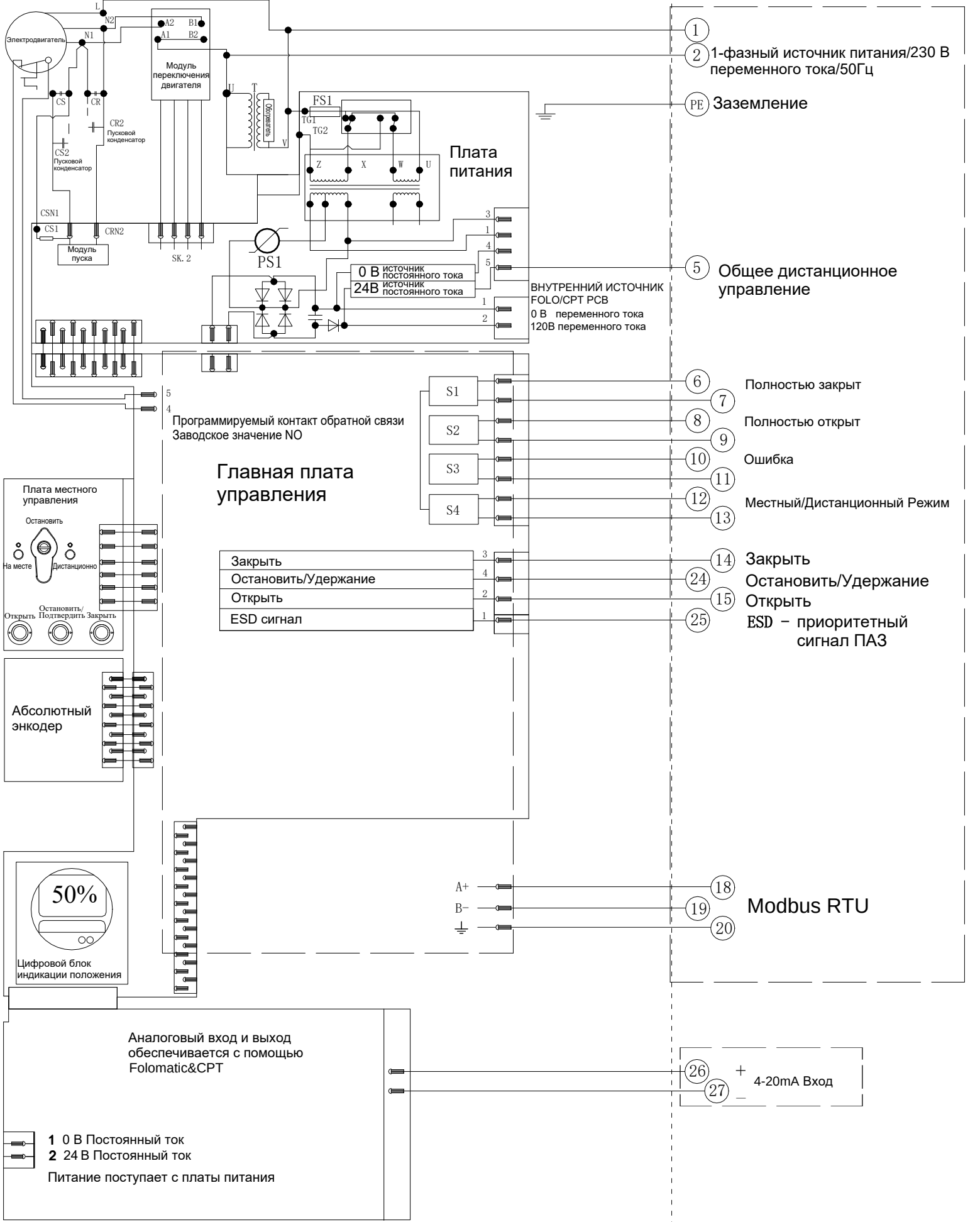
Электрическая схема 4-230-24-4-MR-2 Серия SAL
