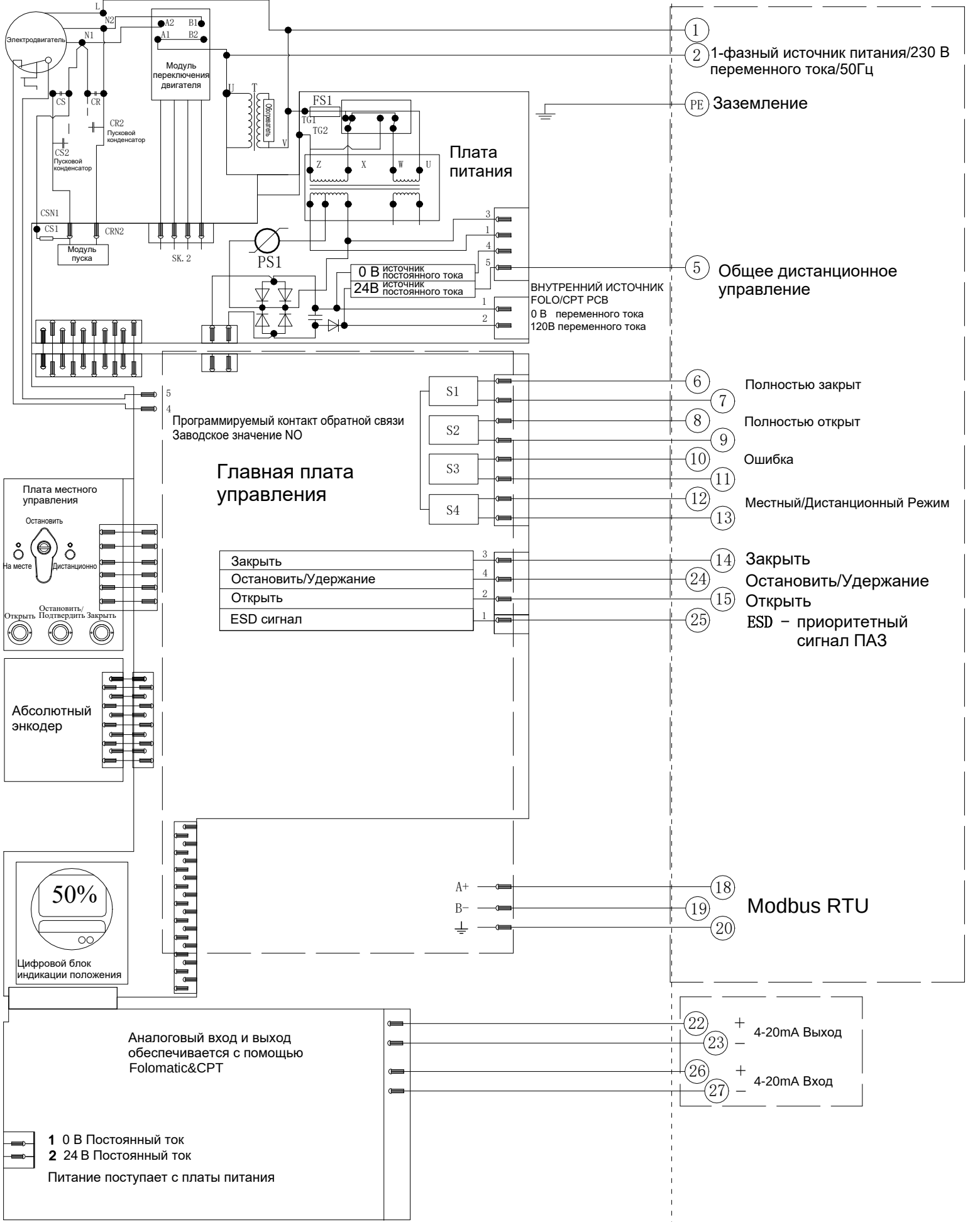
Электрическая схема 4-230-24-4-MR-1 Серия SAL
