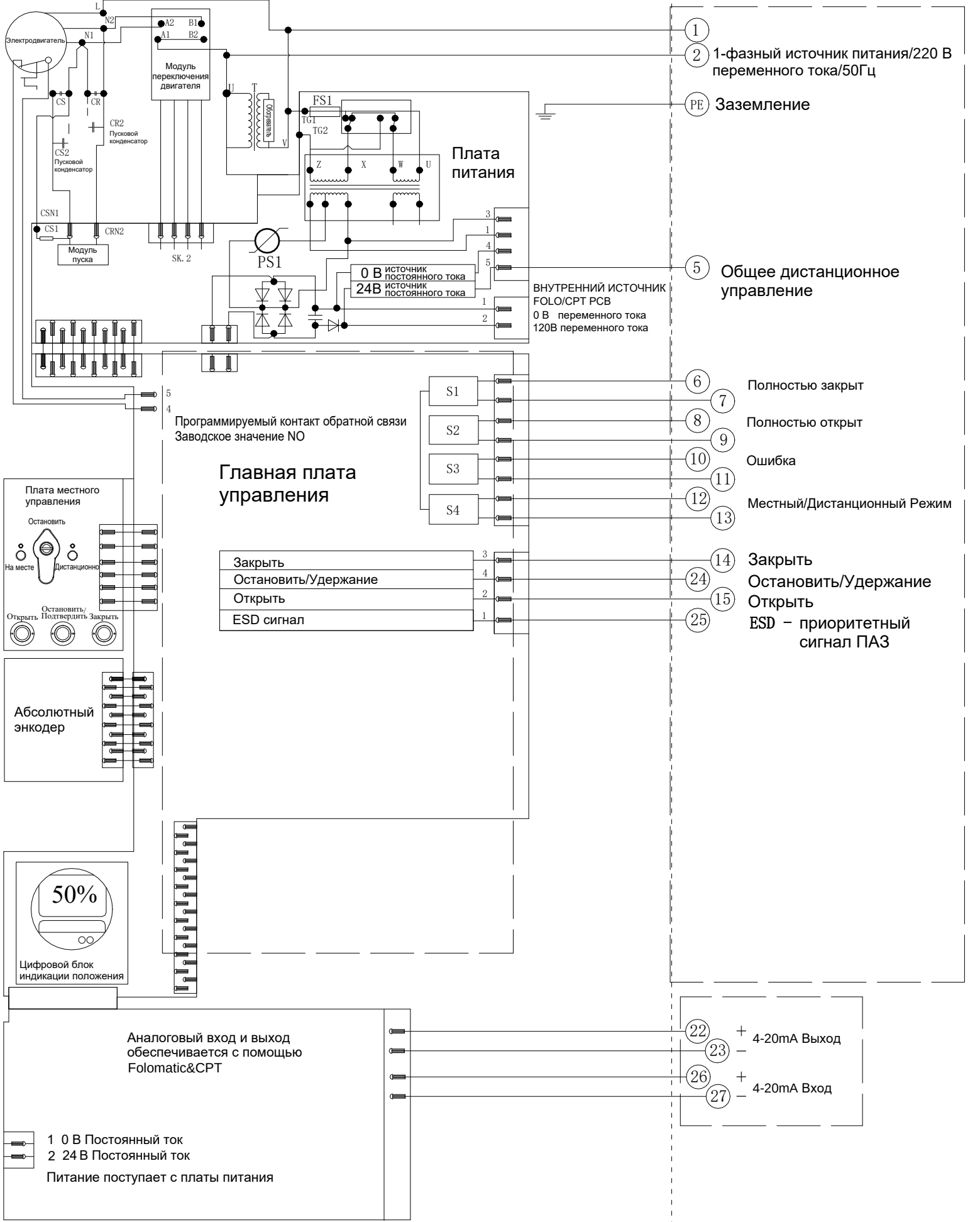
Электрическая схема № 4-220-24-4-N-1 Серия SAL
