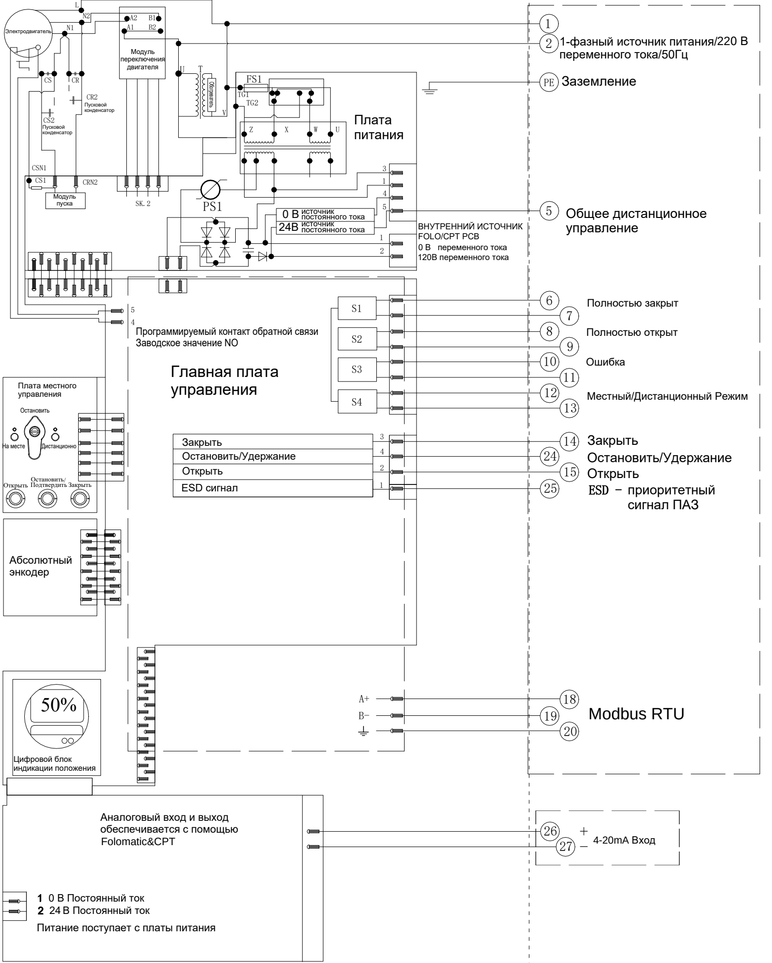
Электрическая схема № 4-220-24-4-MR-2 Серия SAL
