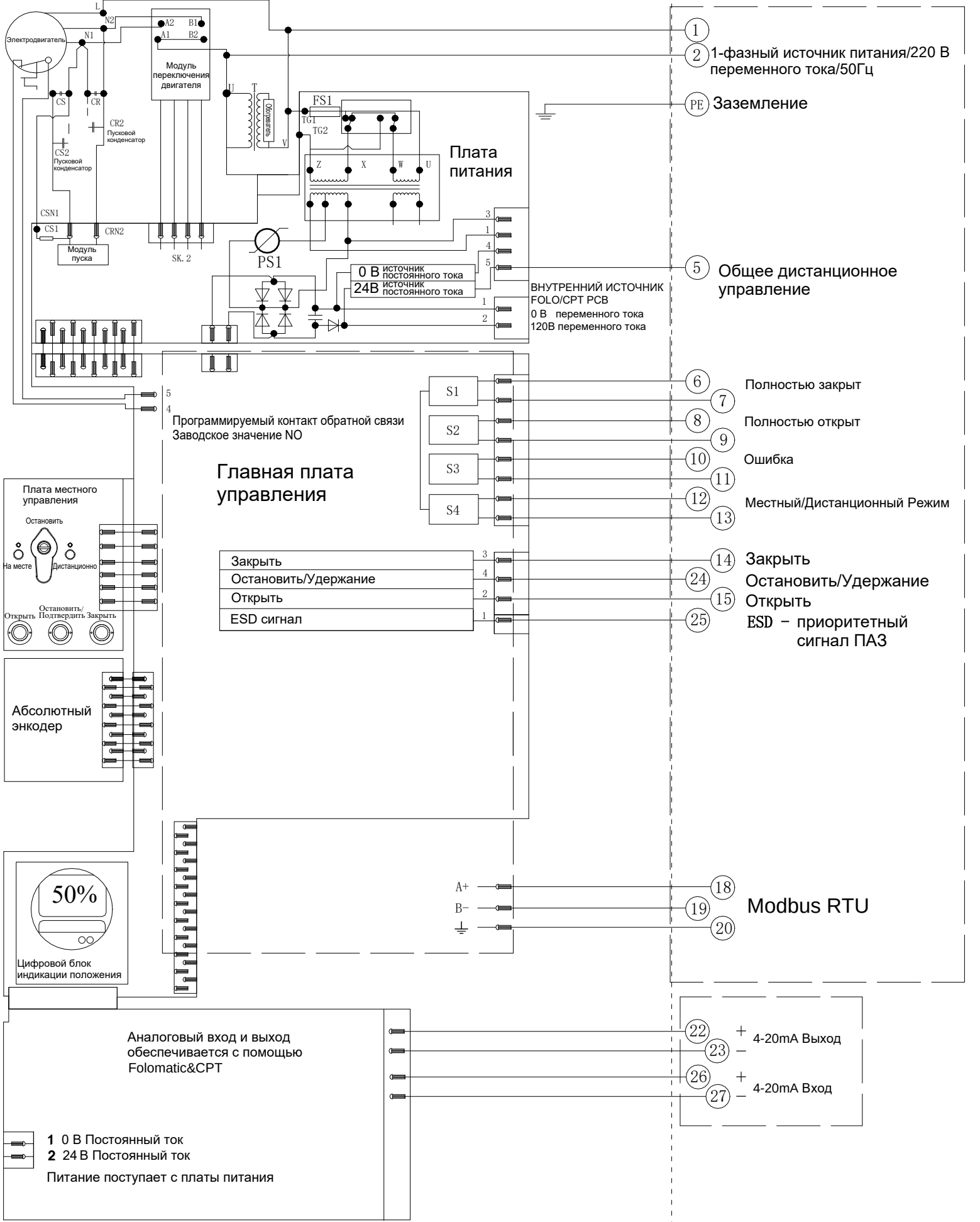
Электрическая схема № 4-220-24-4-MR-1 Серия SAL
