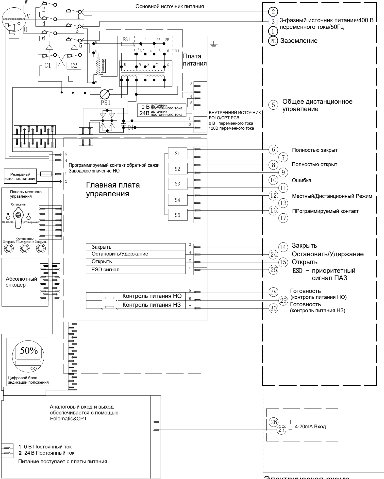
Электрическая схема №8-400В-24-6-N-2 Серия VADQ006-030/100-200
