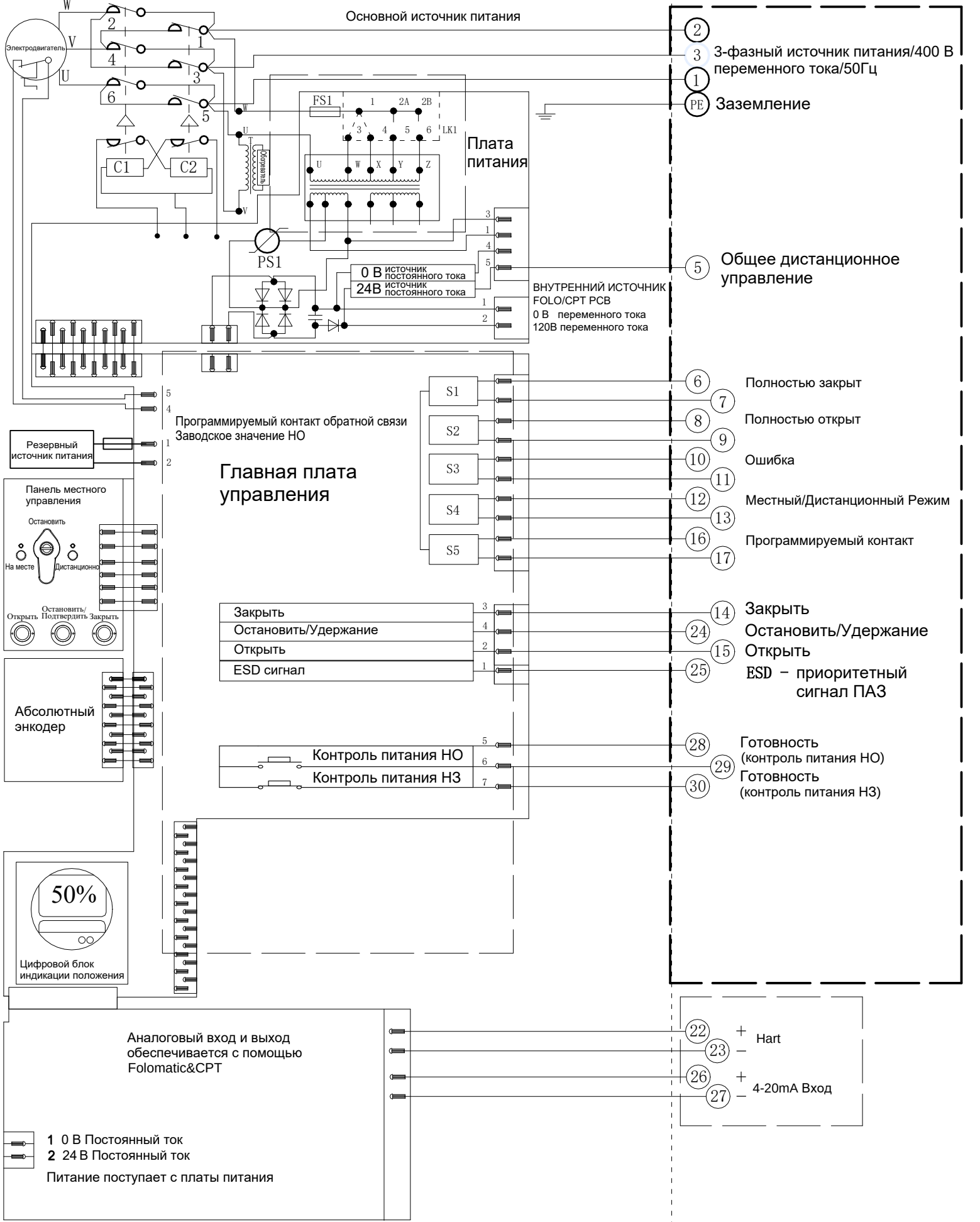
Электрическая схема №8-400В-24-6-HR-2 Серия VADQM006-030/100-200
