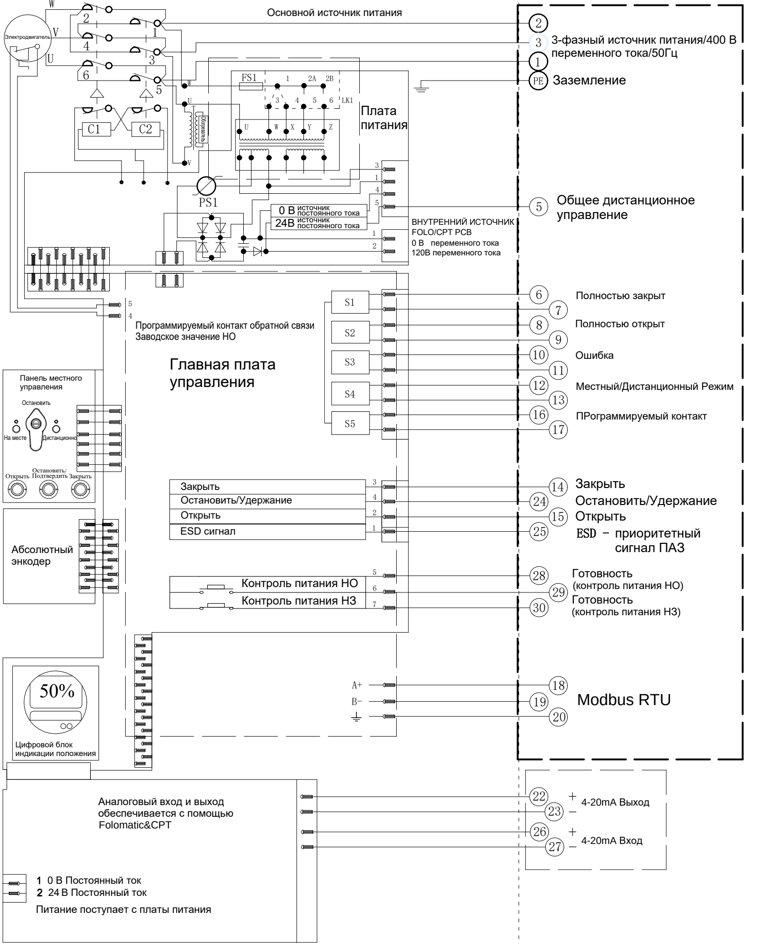
Электрическая схема №8-400-24-6-MR-1 Серия VADQM006-030/100-200
