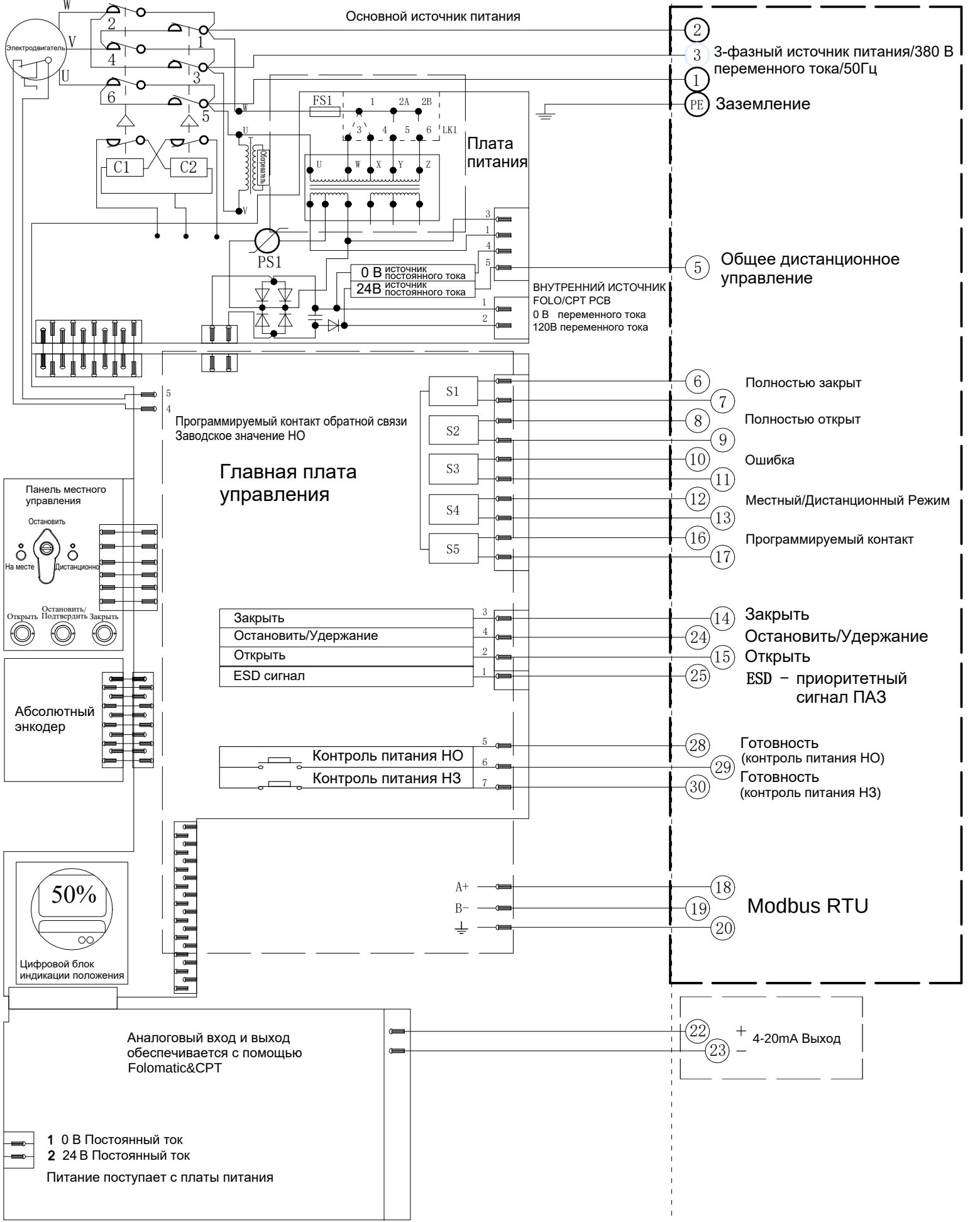
Электрическая схема №8-380-24-6-MR-3 Серия VADQM06-030/100-200
