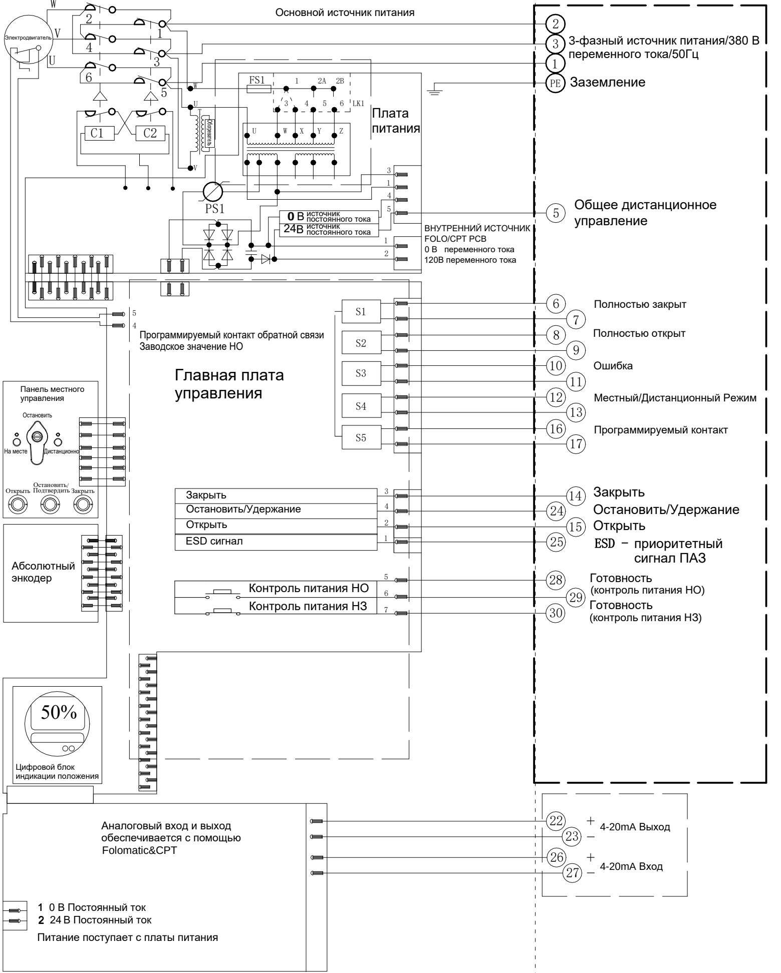
Электрическая схема №8-380-24-6-N-1 Серия VADQM06-030/100-200 Hitewell
