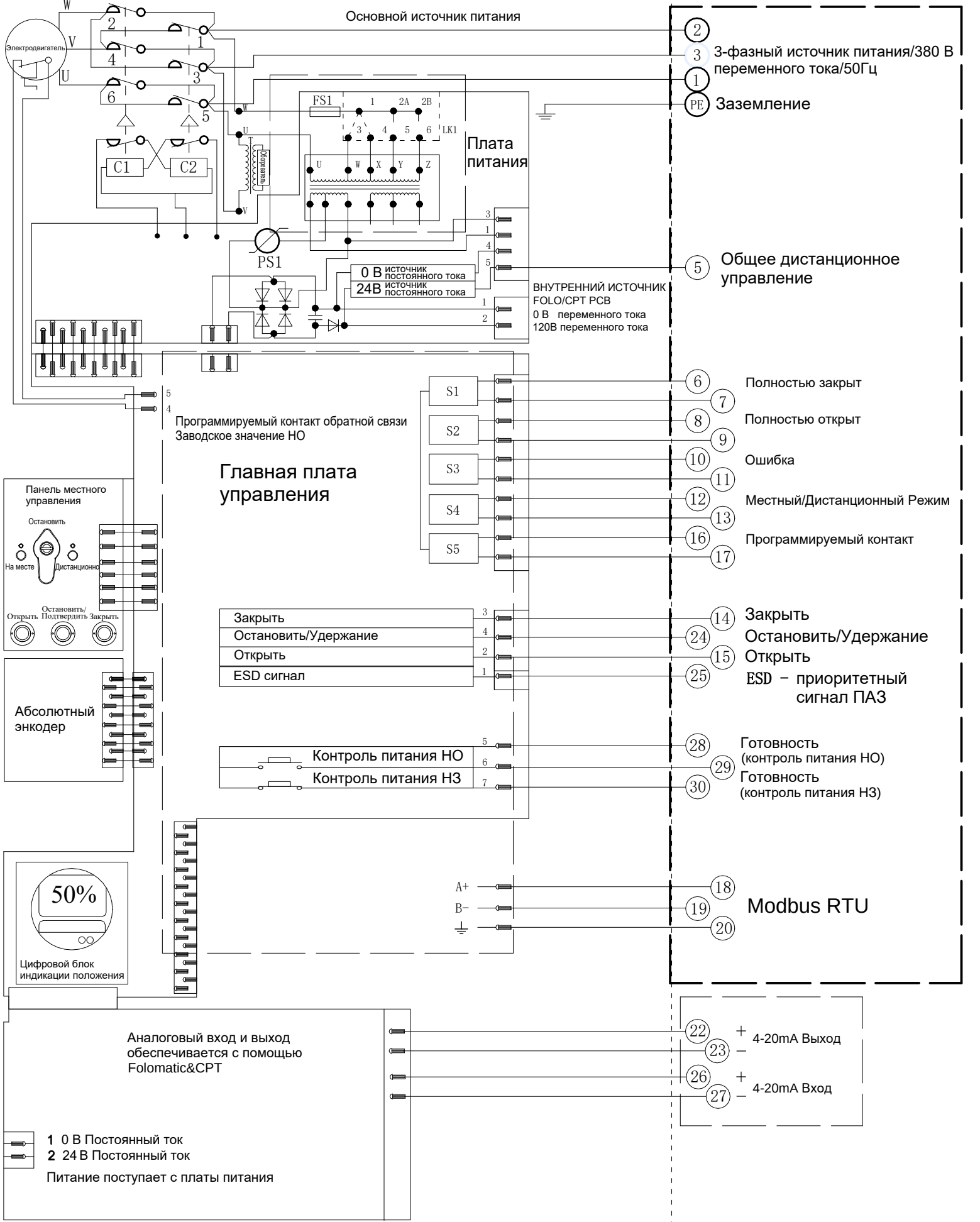
Электрическая схема №8-380-24-6-MR-1 Серия VADQM006-030/100-200
