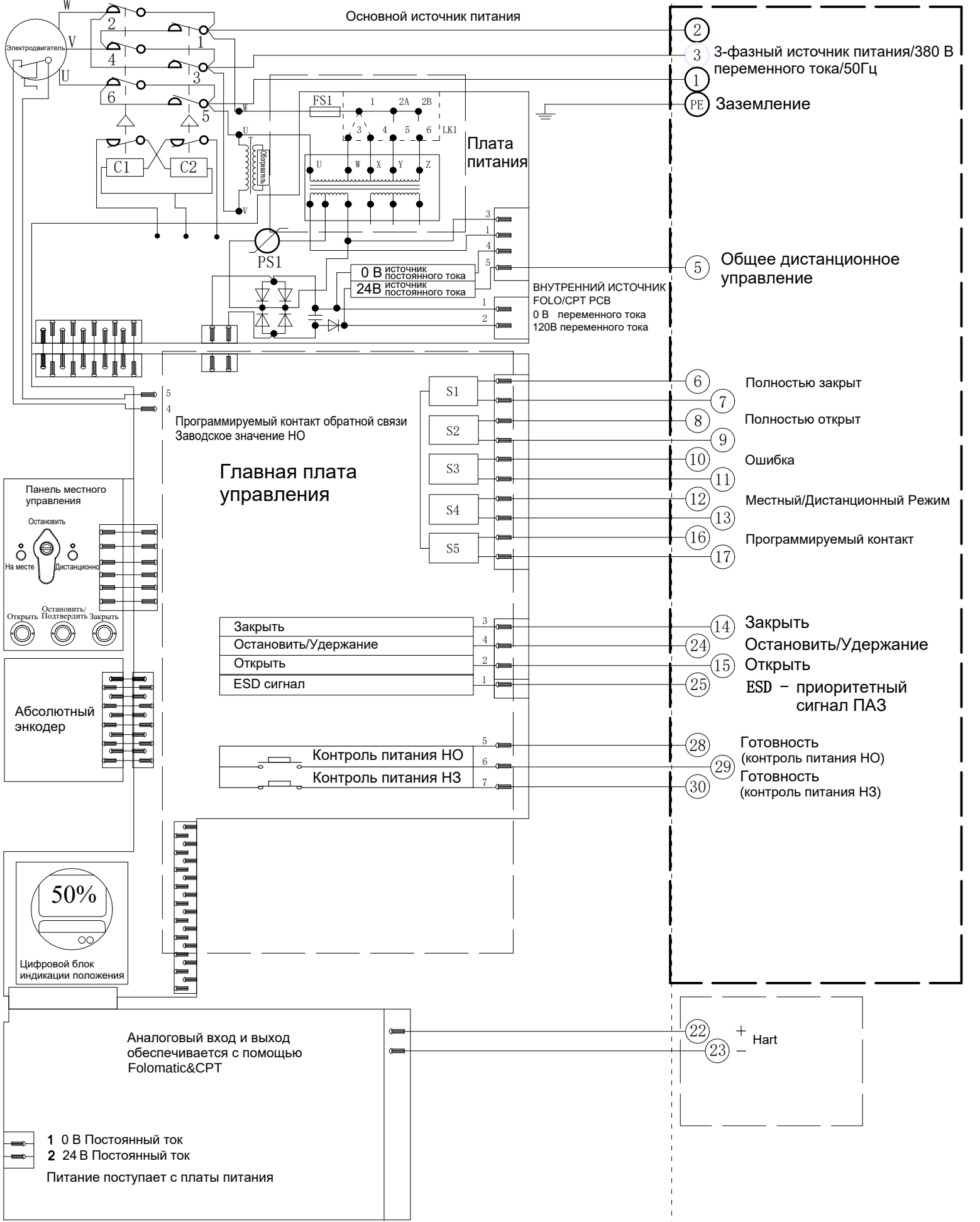
Электрическая схема №8-380-24-6-HR-0 Серия VADQM006-030/100-200
