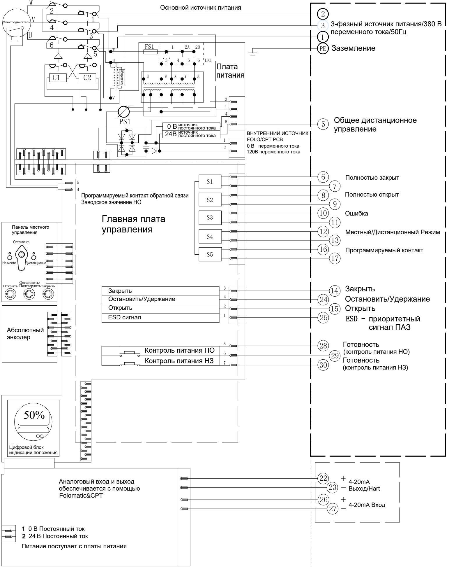
Электрическая схема №8-380-24-6-HR-1 Серия VADQM006-030/100-200
