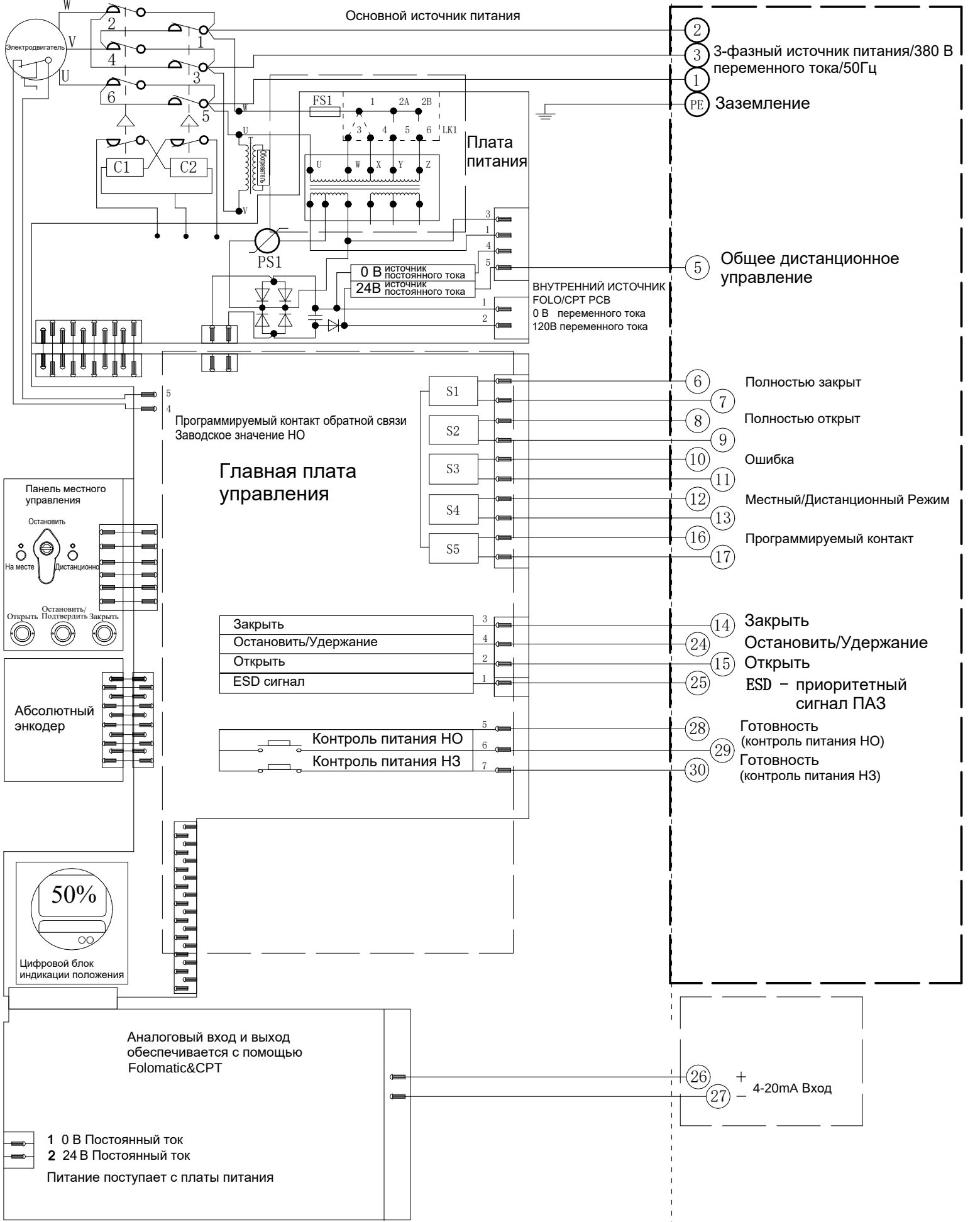
Электрическая схема №8-380-24-6-N-2 Серия VADQM006-030/100-200
