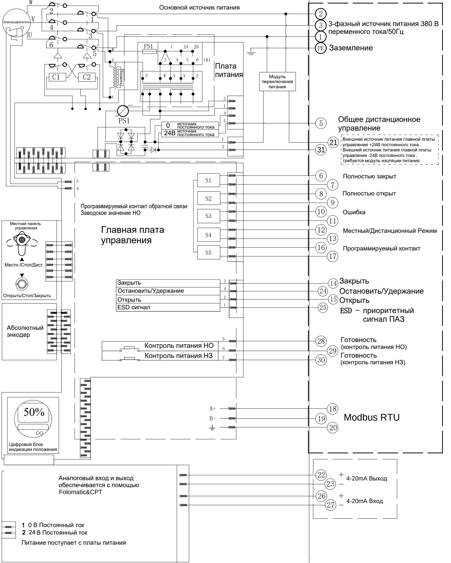
Электрическая схема №8-380A-24-6-MR-1 Серия VADQM006-030/100-200
