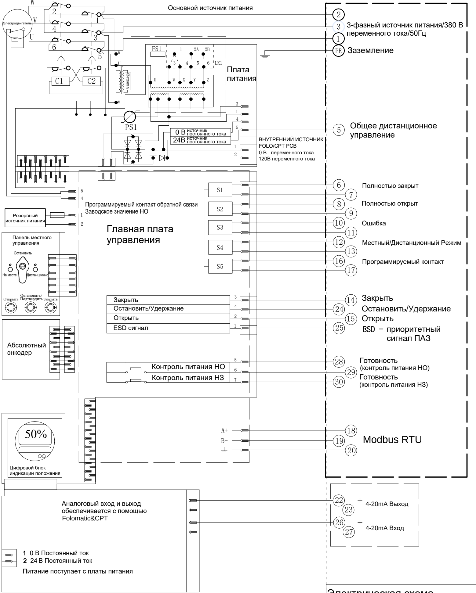
Электрическая схема №8-380В-24-6-MR-1 Серия VADQM006-030/100-200
