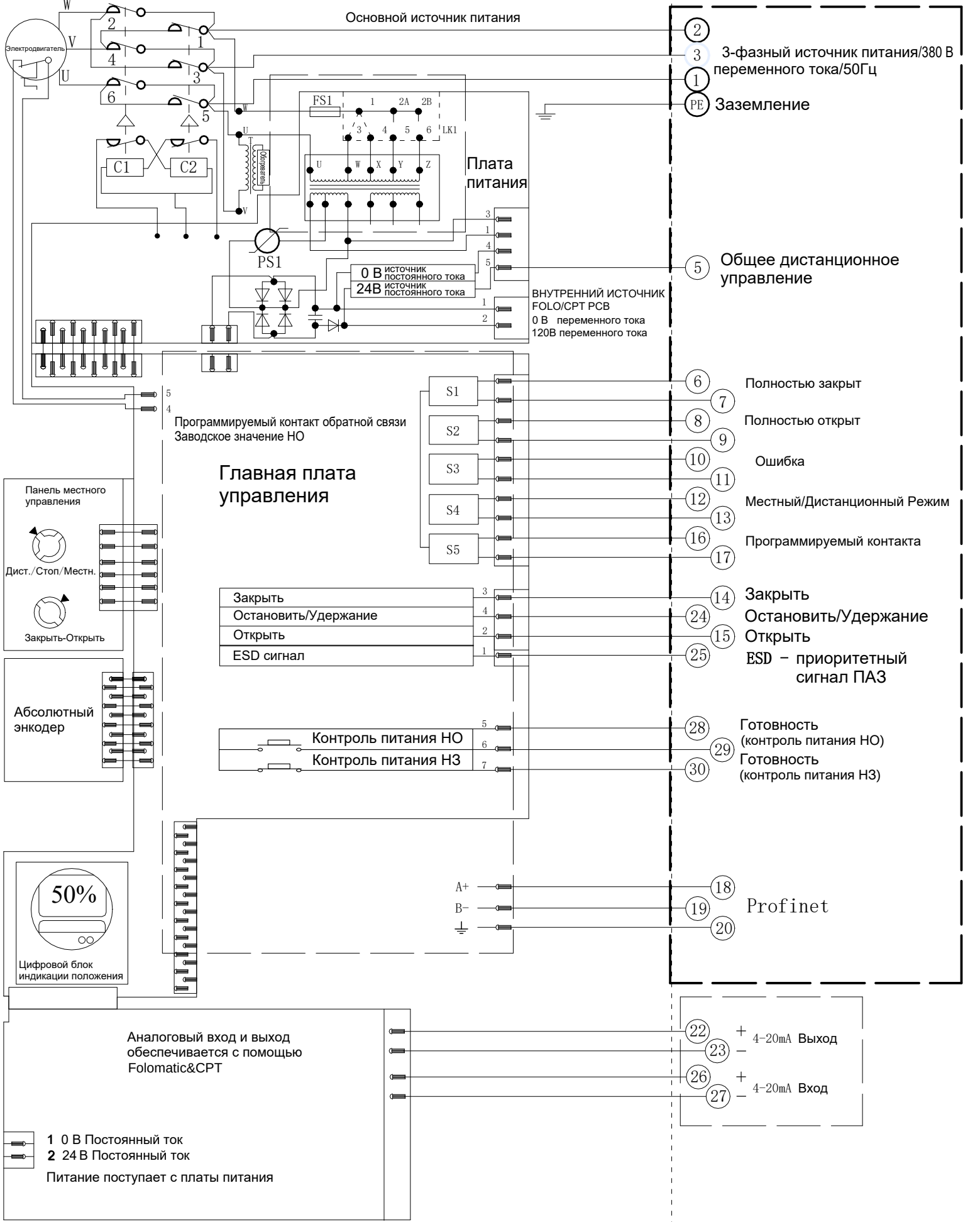
Электрическая схема: № 8-380-24-6-PN-1 Серия VADQM006-030/100-200
