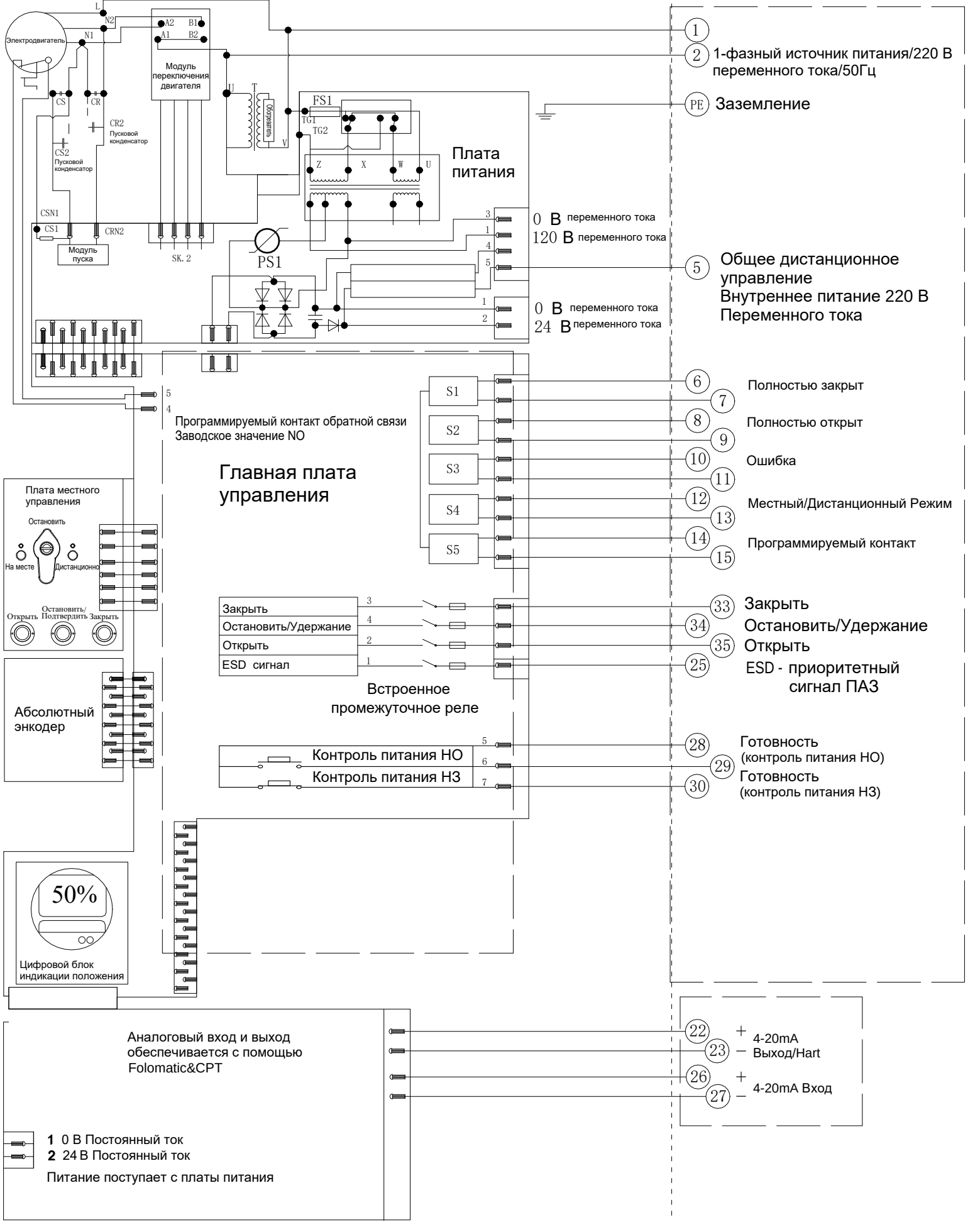
Электрическая схема №8-220-220-6-HR-1 Серия VADQM006-030-100-200
