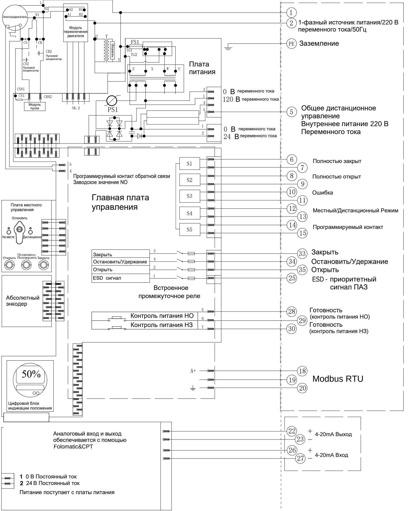
Электрическая схема №8-220-220-6-MR- 1 Серия VADQM006-030/100-200
