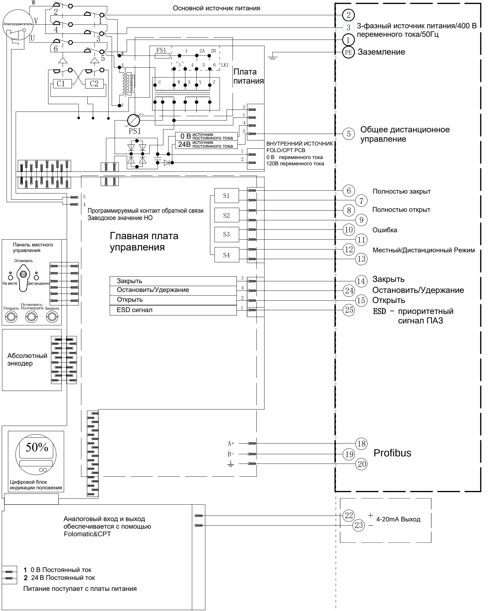
Электрическая схема №8-400-24-4-PR-3 Серия VADQM006-030/100-200
