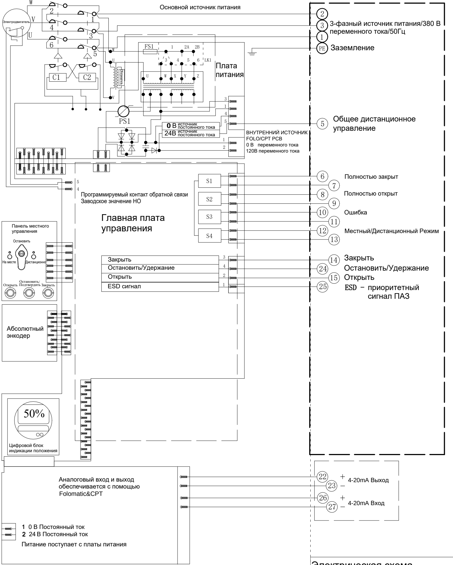
Электрическая схема №8-380-24-4-N-1 Серия VADQM006-030/100-200
